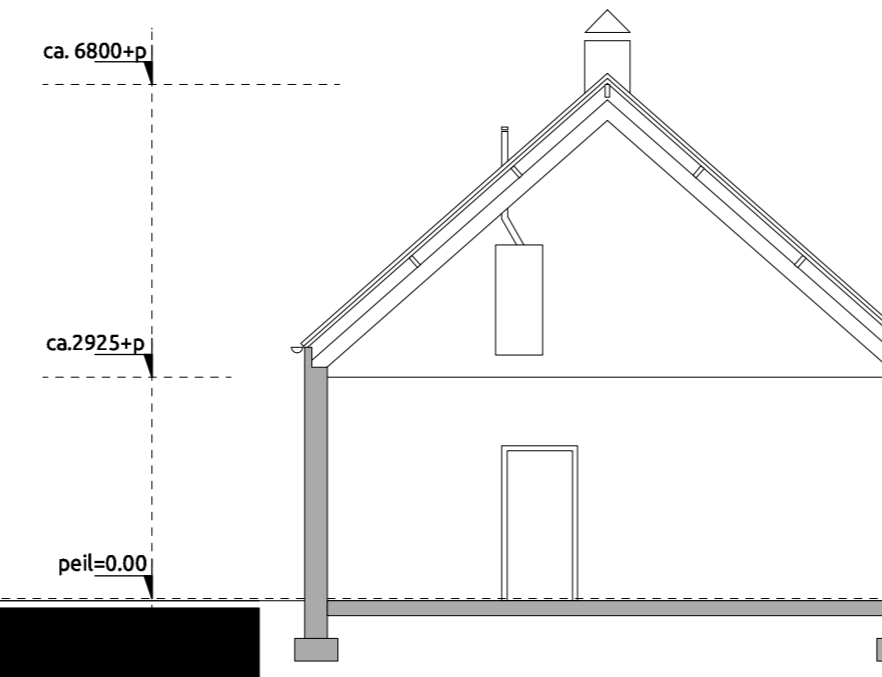
doorsnede A-A
