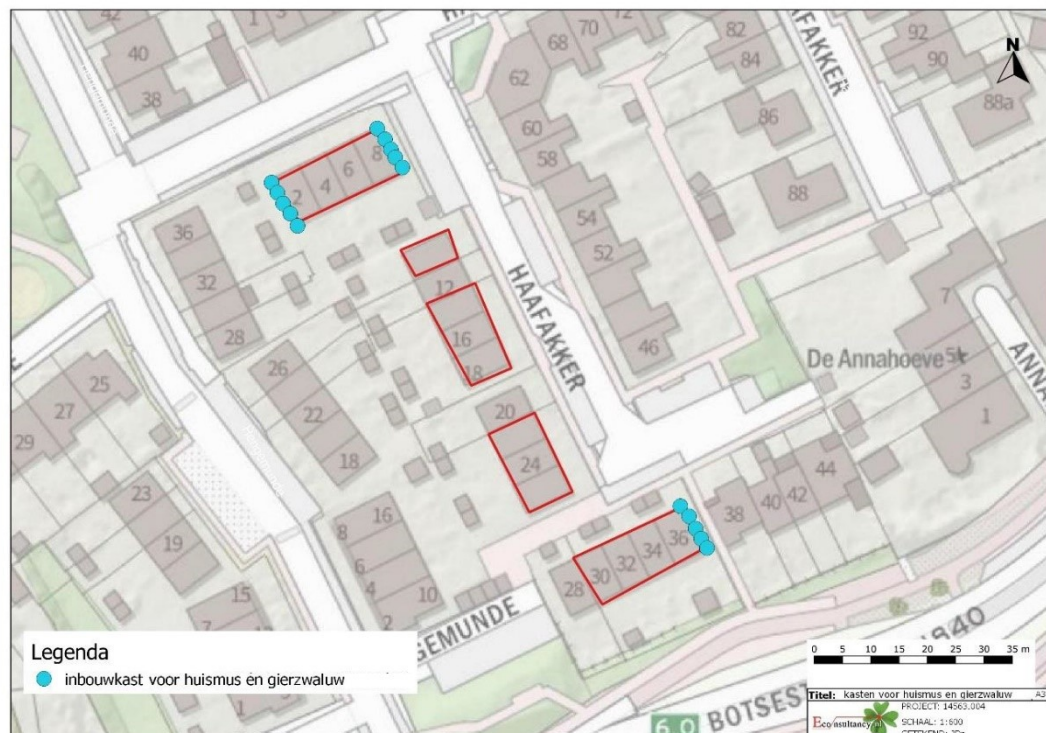
Figuur 4. Locaties inbouwkasten voor de huismus en de gierzwaluw (10 voor de huismus en 5 voor de gierzwaluw).
