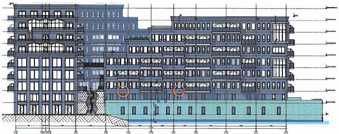
Figuur 2: Inbouwkasten voor vleermuizen in de achtergevel/westergevel (een per cirkel).
