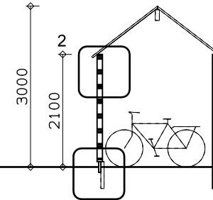
Doorsnede
