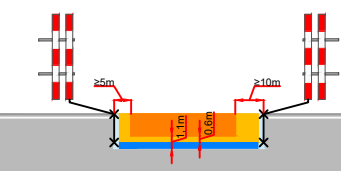
Werkvakindeling ETW
