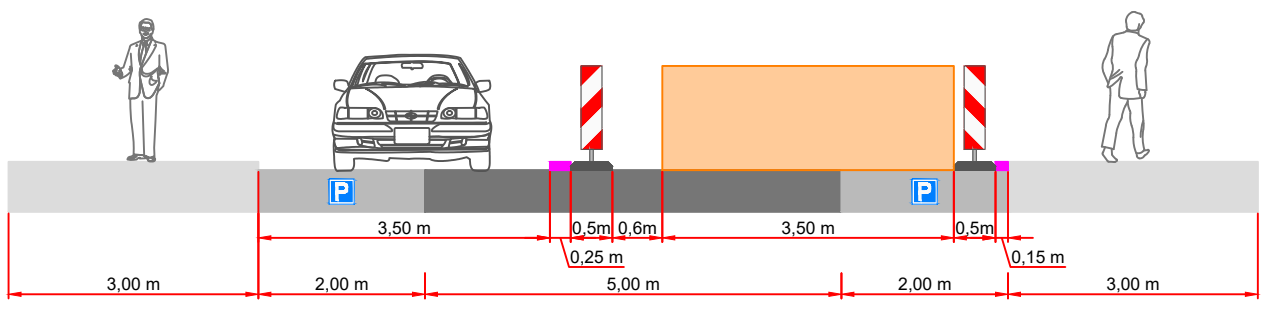
Dwarsdoorsnede C-C
