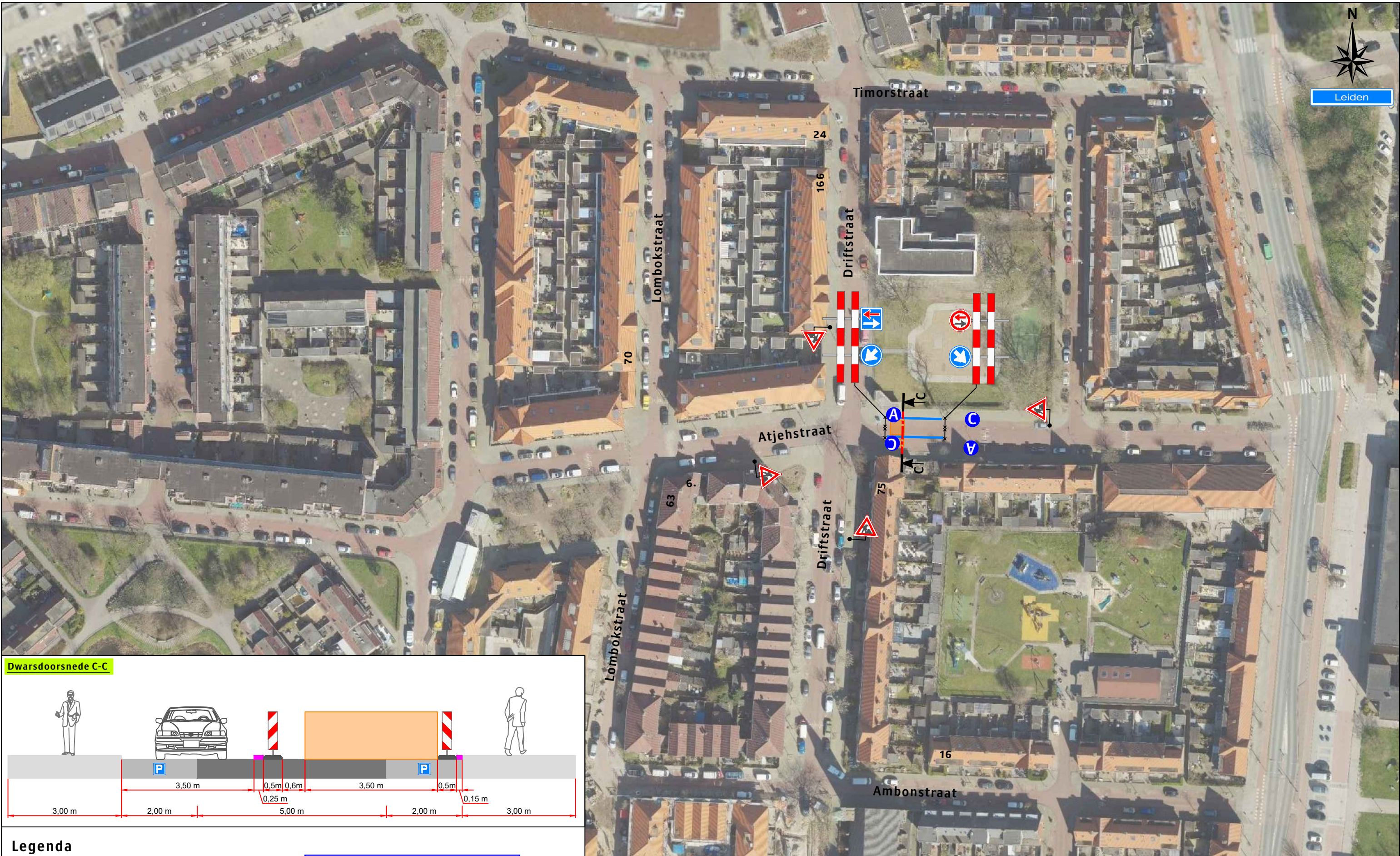
Werkvakindeling ETW
