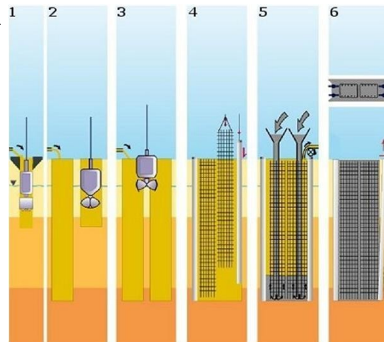
Diepwand (aanlegmethode)
