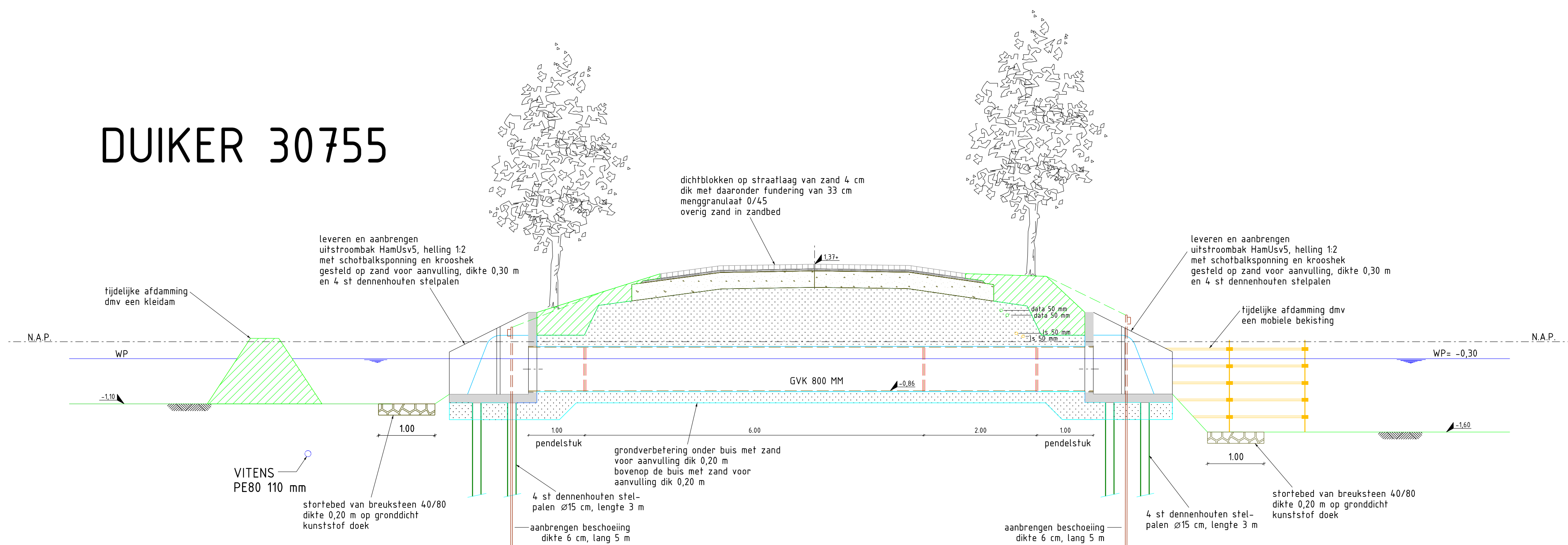
DOORSNEDE A-A SCHAAL 1:50
