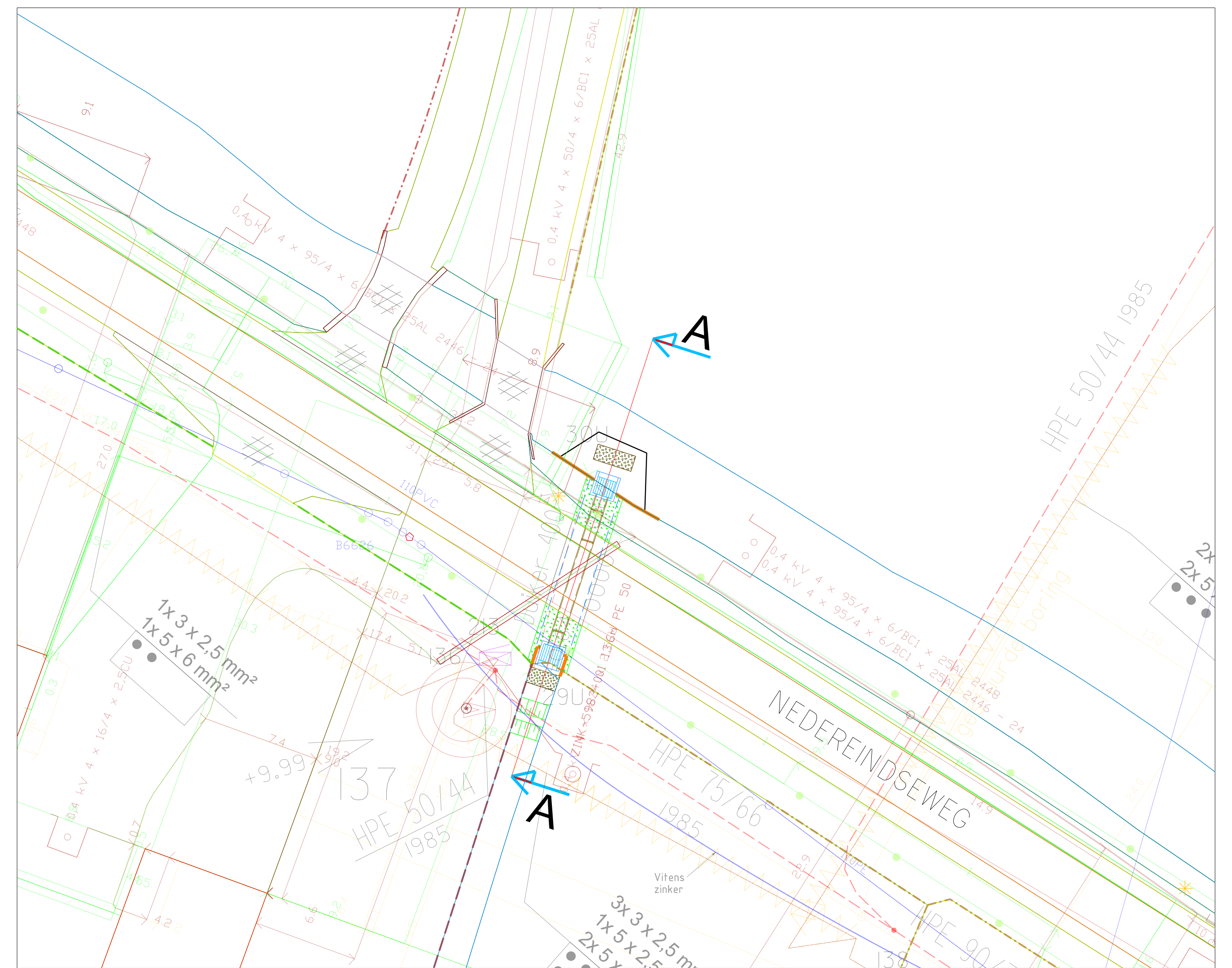
DOORSNEDE DUIKER MET KABELS EN LEIDINGEN schaal 1:200
