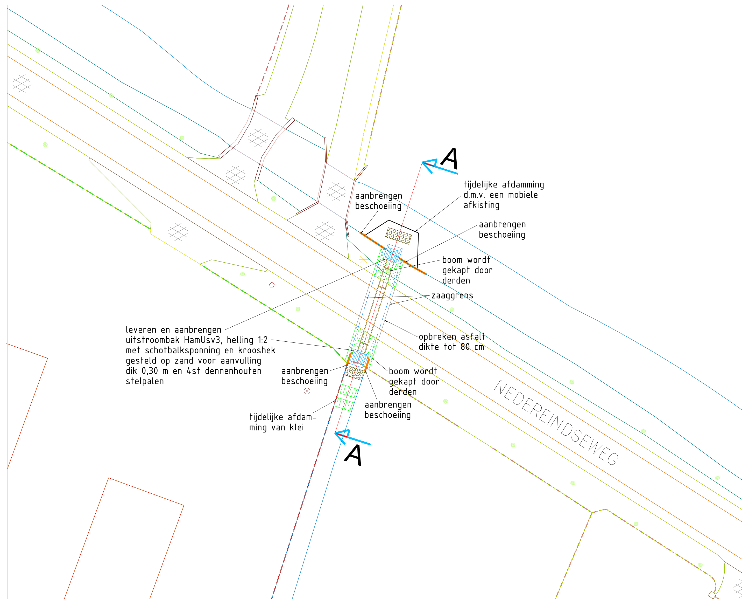
NIEUWE SITUATIE DUIKER schaal 1:200
