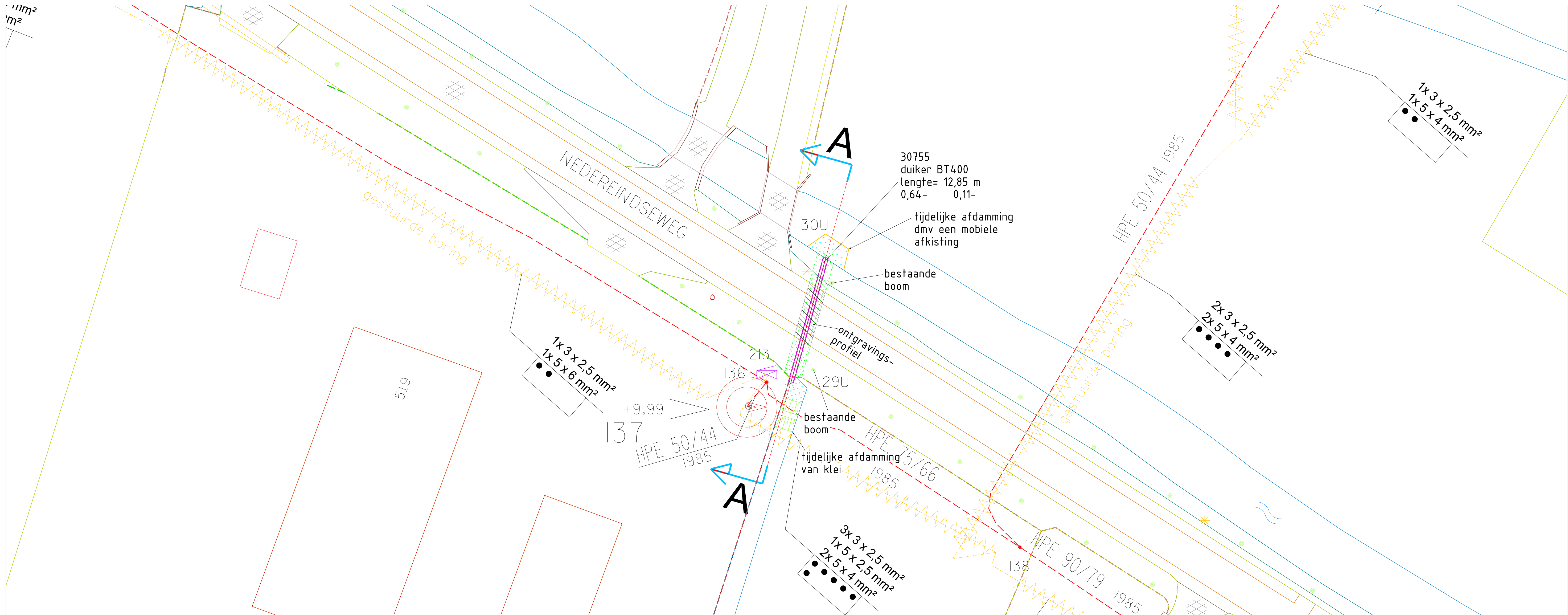
BESTAANDE SITUATIE schaal 1:200
