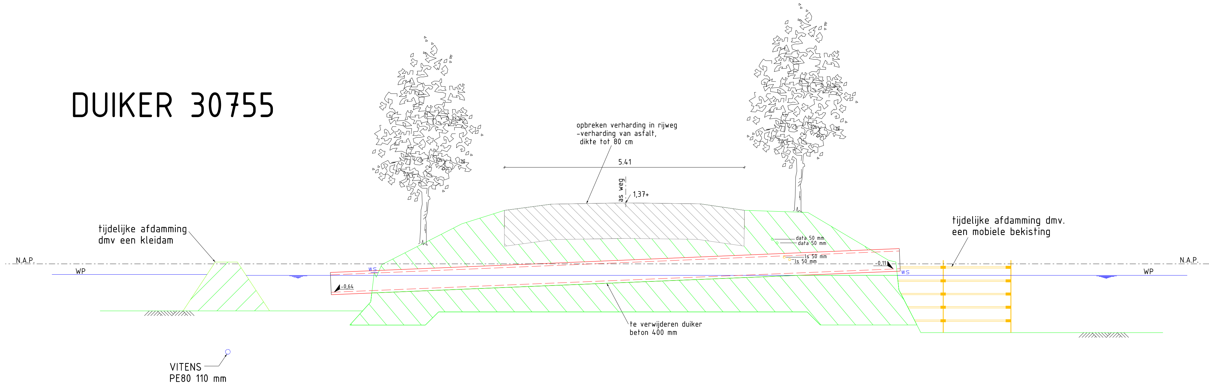
DOORSNEDE A-A SCHAAL 1:50
