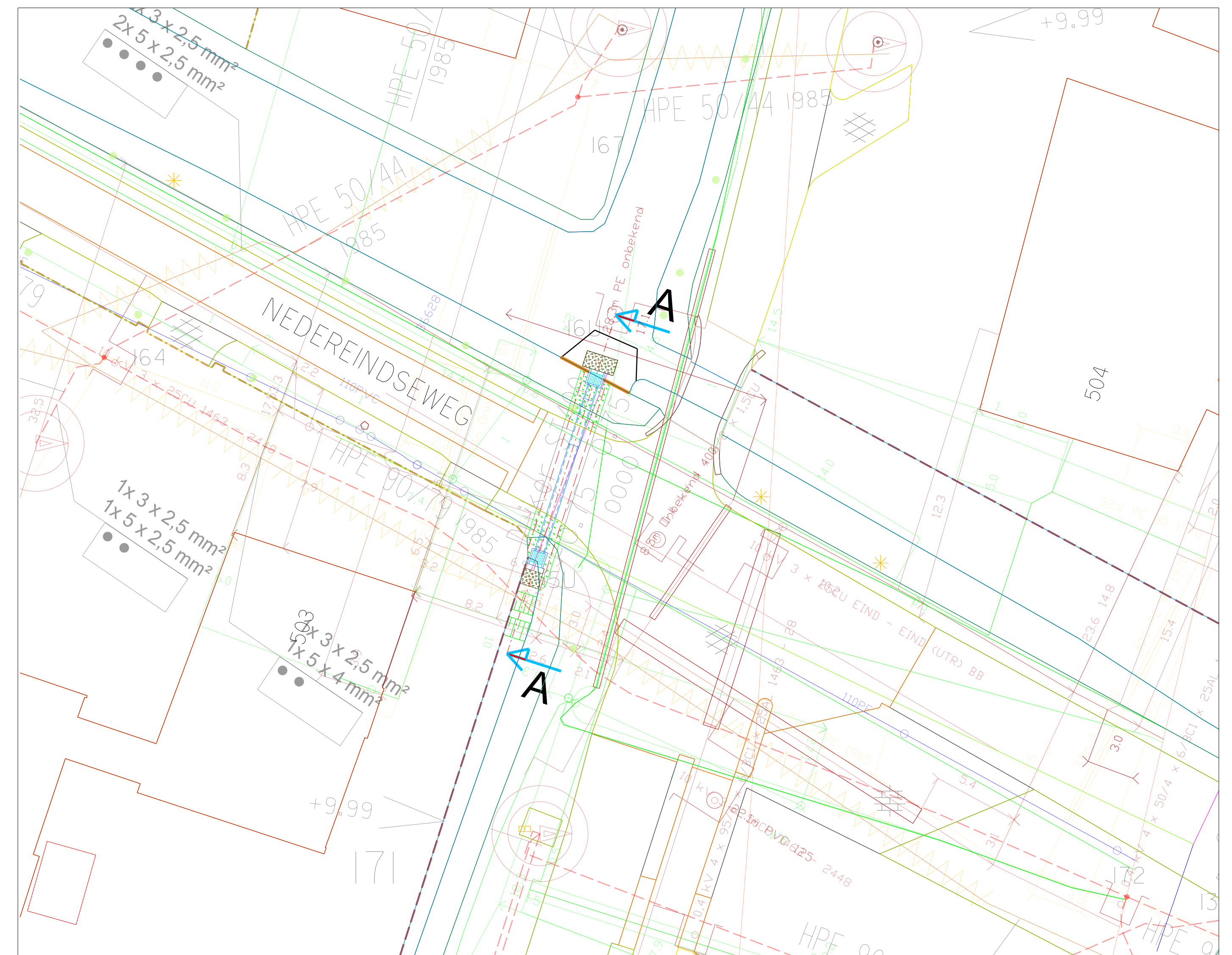
NIEUWE SITUATIE DUIKER MET KABELS EN LEIDINGEN schaal 1:200
