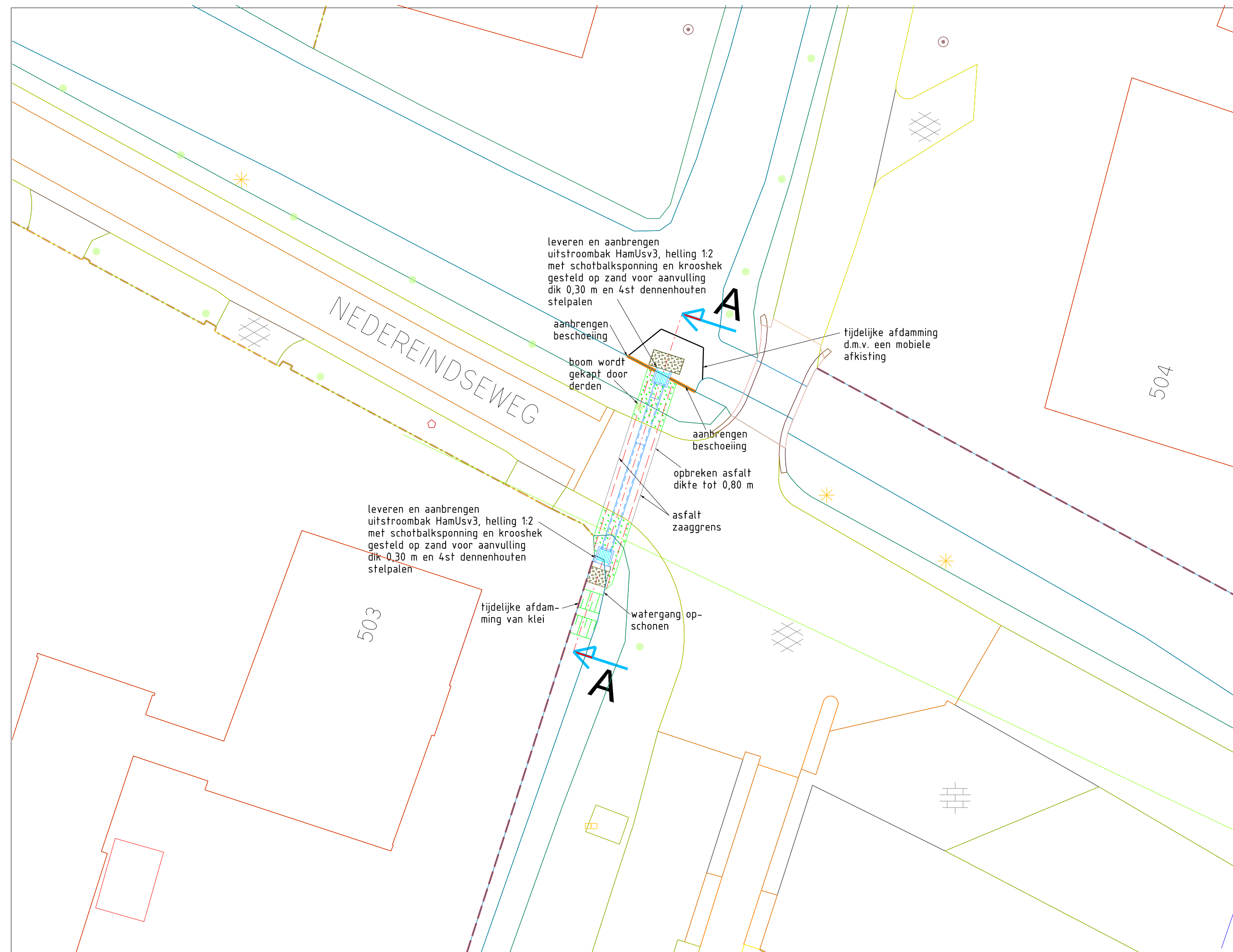
NIEUWE SITUATIE DUIKER schaal 1:200
