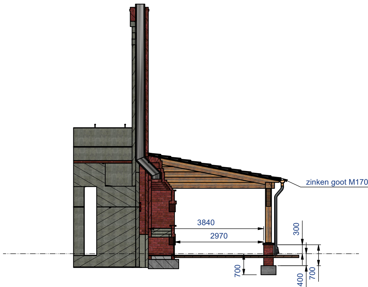
A-A ( 1 :75 )
