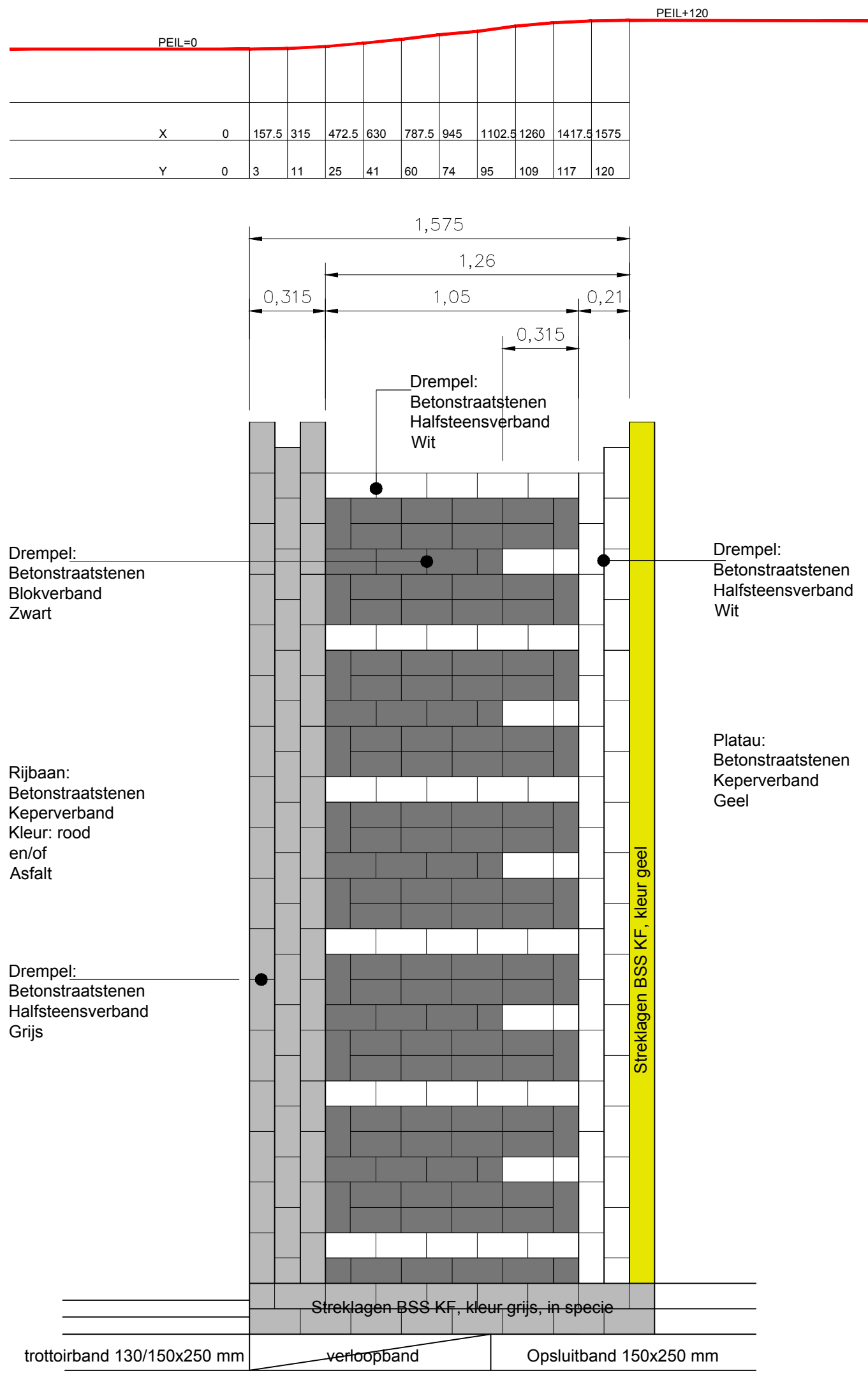
Principedetail 30 km/h talud plateau Schaal 1:20
