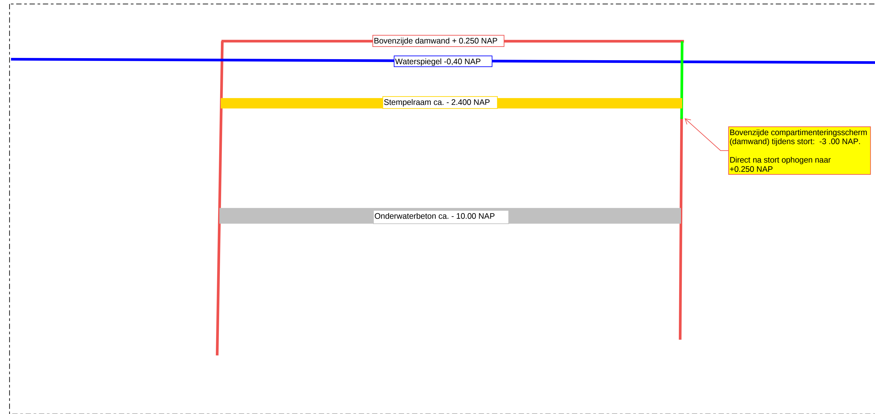
Doorsnede / Situatie tekening t.b.v. storten OnderWaterBeton compartiment 1 (weekend van week 44/45-2021), en compartiment 2 (weekend van week 50/51-2021).
