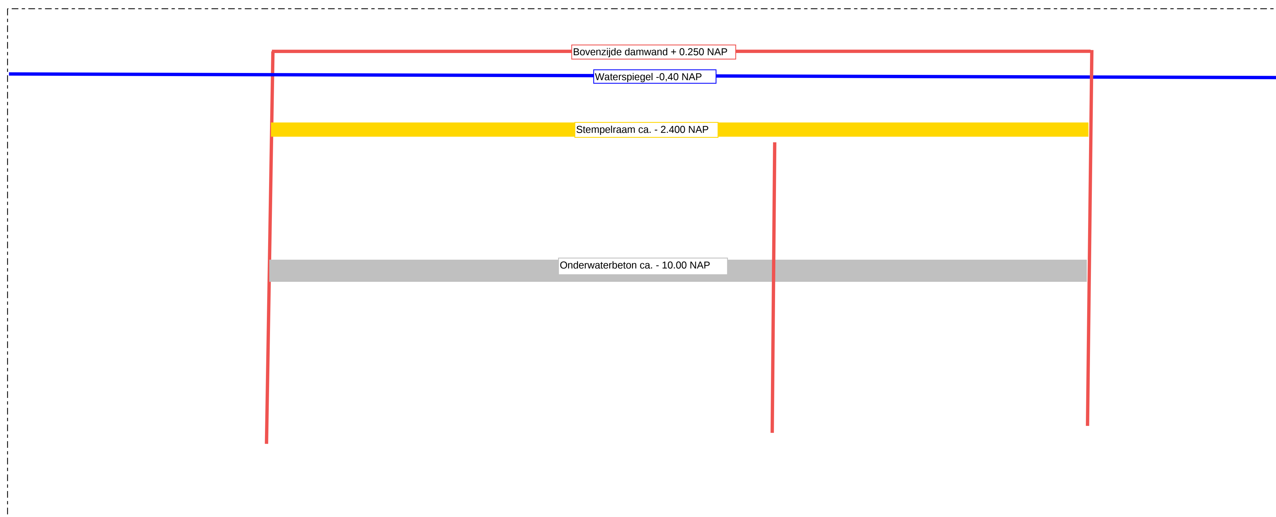
Doorsnede / Situatie tekening t.b.v. storten OnderWaterBeton compartiment 3 en 4 (weekend van week 6/7-2022).
