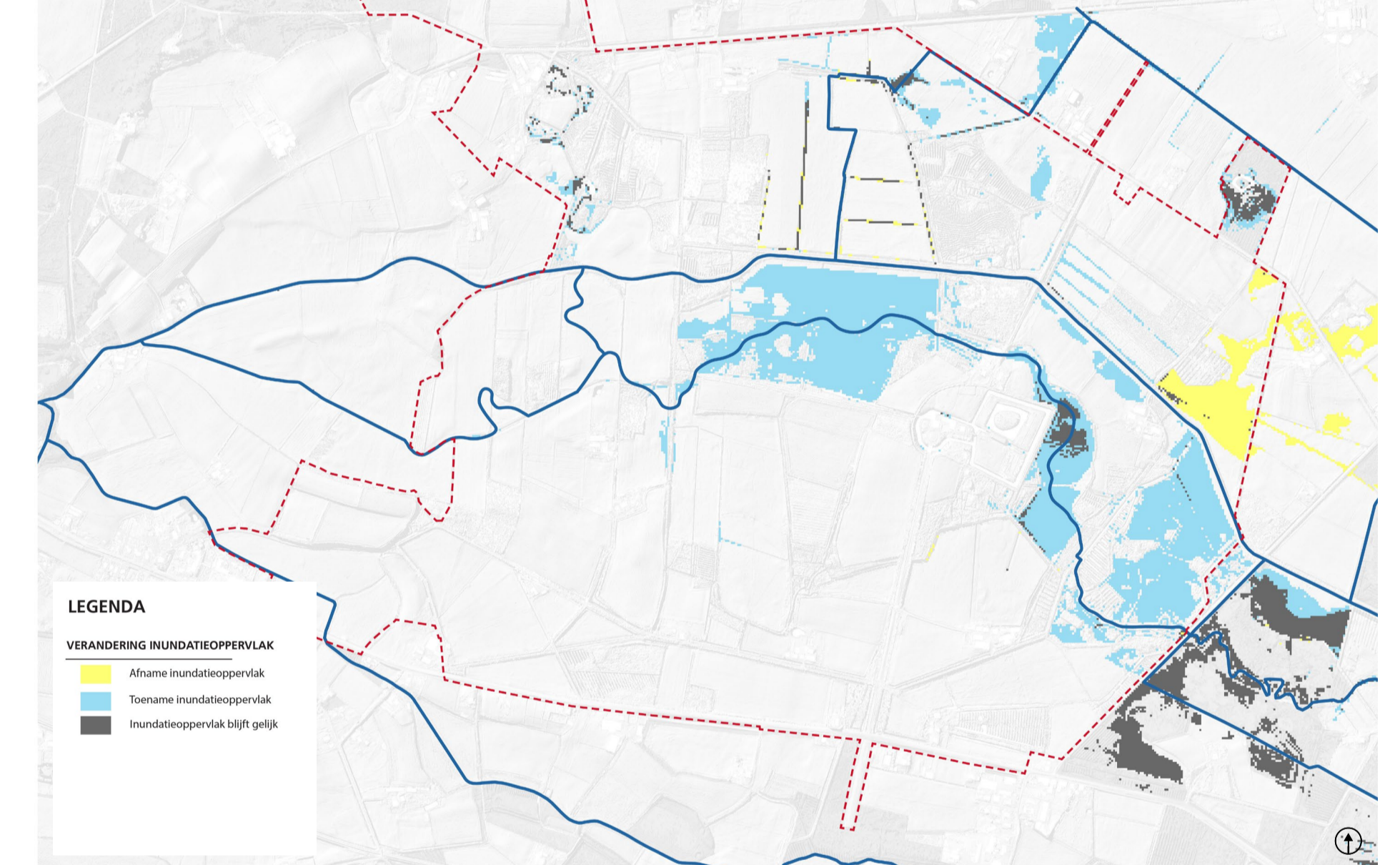
VERANDERING INUNDATIEOPPERVLAK T=10
