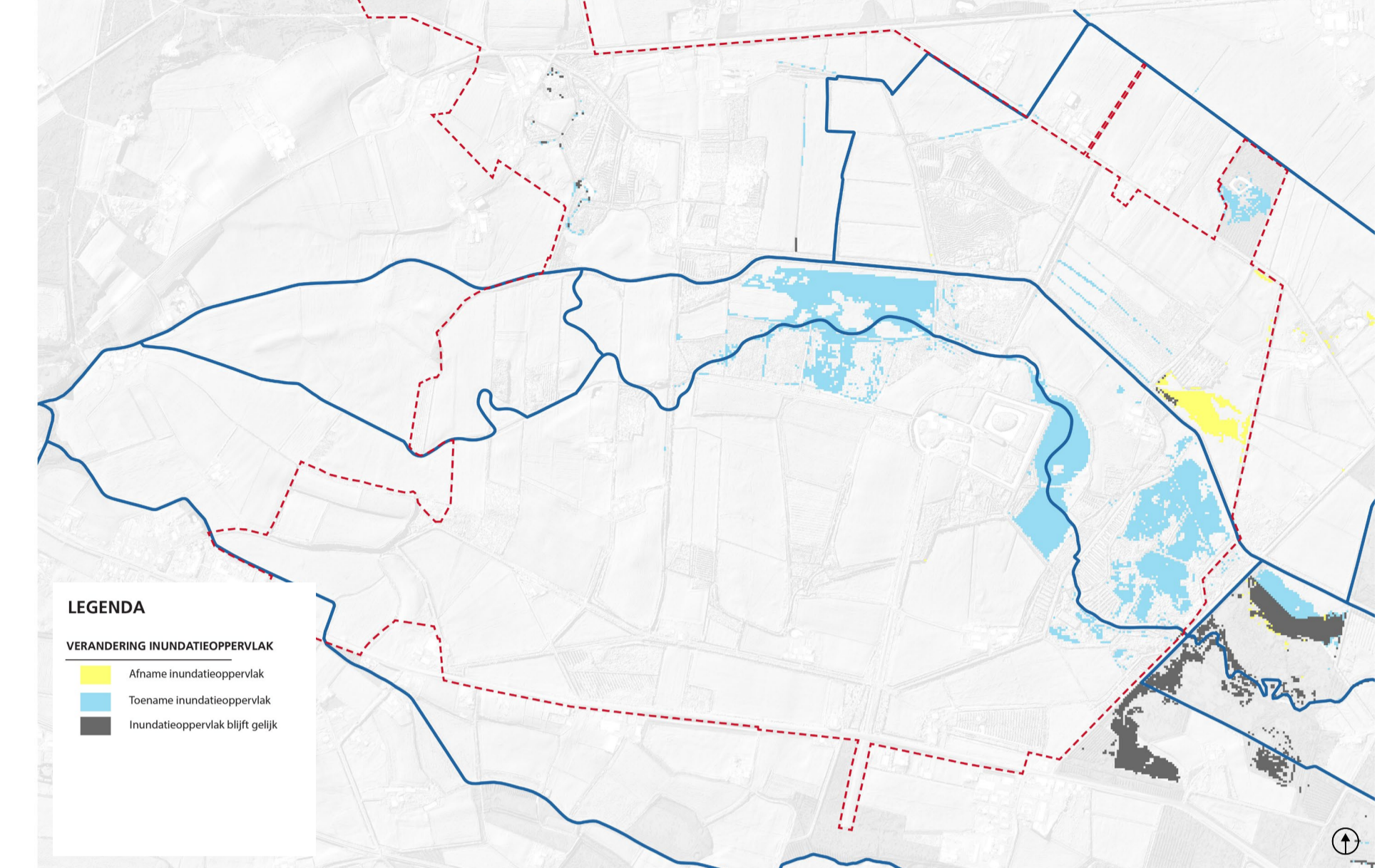
VERANDERING INUNDATIEOPPERVLAK T=1
