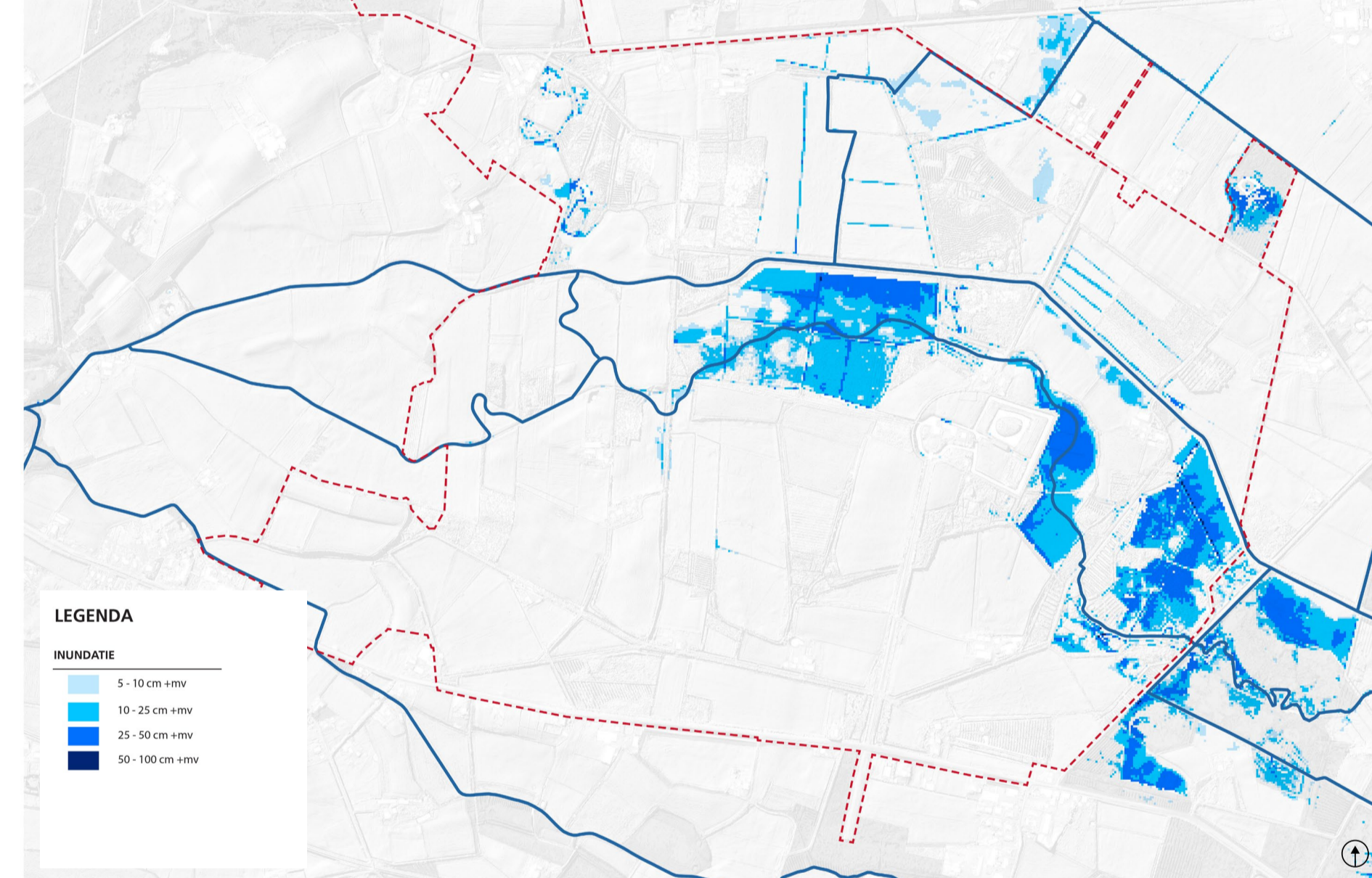
DO - INUNDATIE T=10
