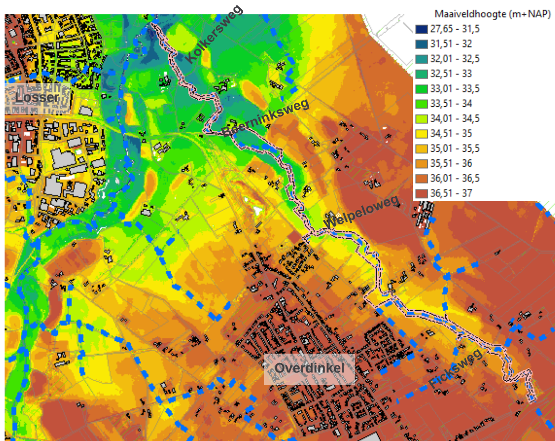
Figuur 2.3 Maaiveldhoogteverloop langs de Ruhenbergerbeek met de leggerwaterlopen (blauw gesitpeld, roze omlijnd is projectgebied)
