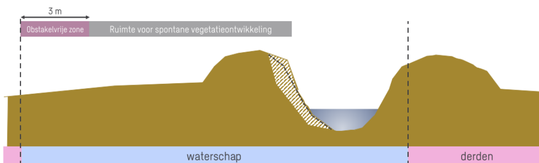
Figuur 4.1 Schematische weergave maatregel puin verwijderen
