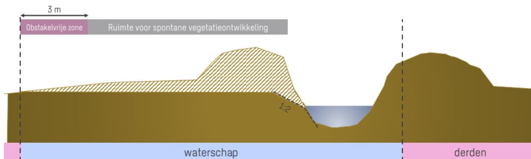
Figuur 4.2 Schematische weergave maatregel verwijderen kunstmatige wal
