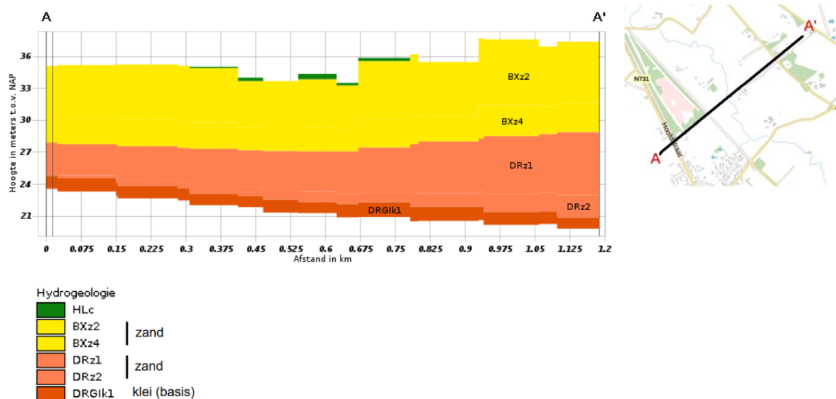
Figuur 2.2 Geohydrologische opbouw beekdal en omgeving Ruhenbergerbeek
