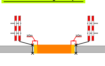
Werkvakindeling voetpad
