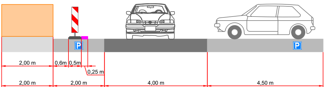
Werkvakindeling voetpad
