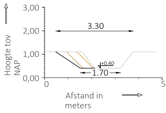
Varelsebeek, profiel 1 Schaal 1:100
