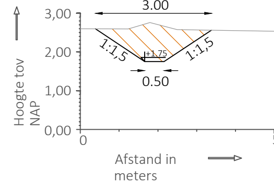
Randsloot 1, profiel 6 Schaal 1:100
