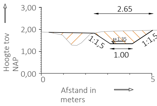
Randsloot 2, profiel 3 Schaal 1:100
