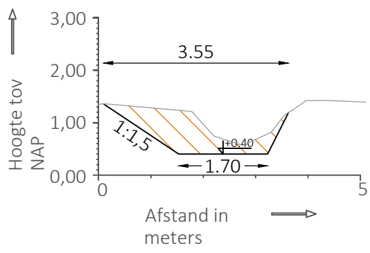
Randsloot 2, profiel 2a Schaal 1:100
