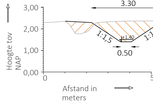
Randsloot 1, profiel 5 Schaal 1:100
