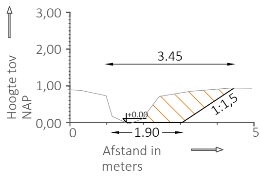
Randsloot 2, profiel 1 Schaal 1:100
