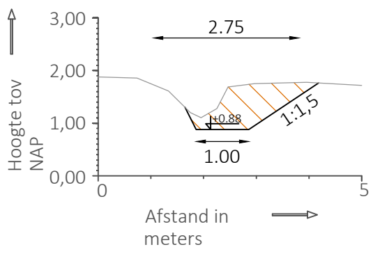
Randsloot 2, profiel 2b Schaal 1:100
