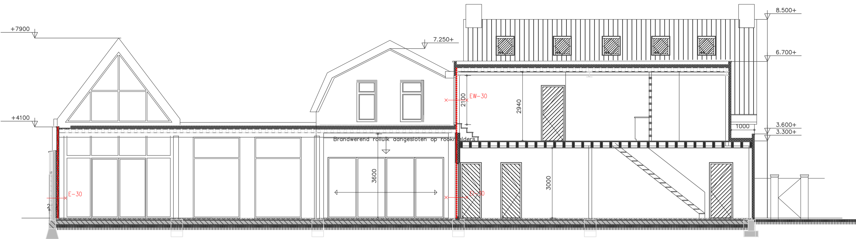
Doorsnede AA
