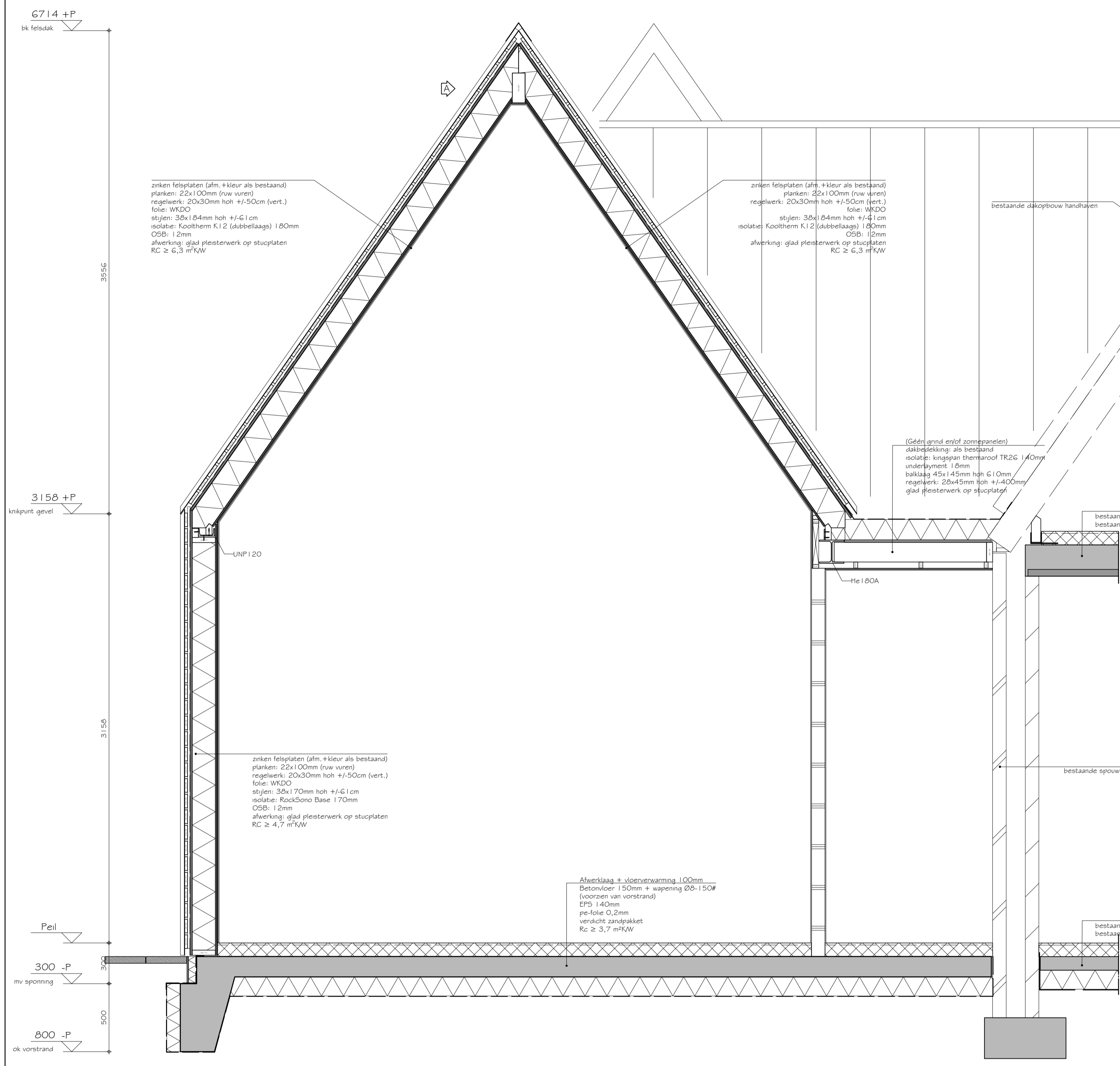
DOORSNEDE A-A
