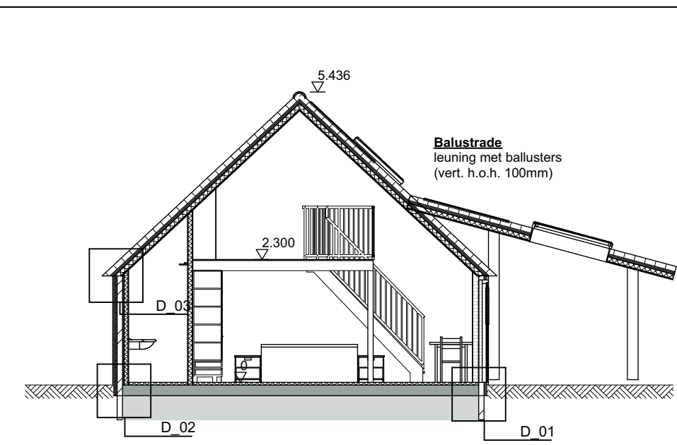
Doorsnede B1-B1
