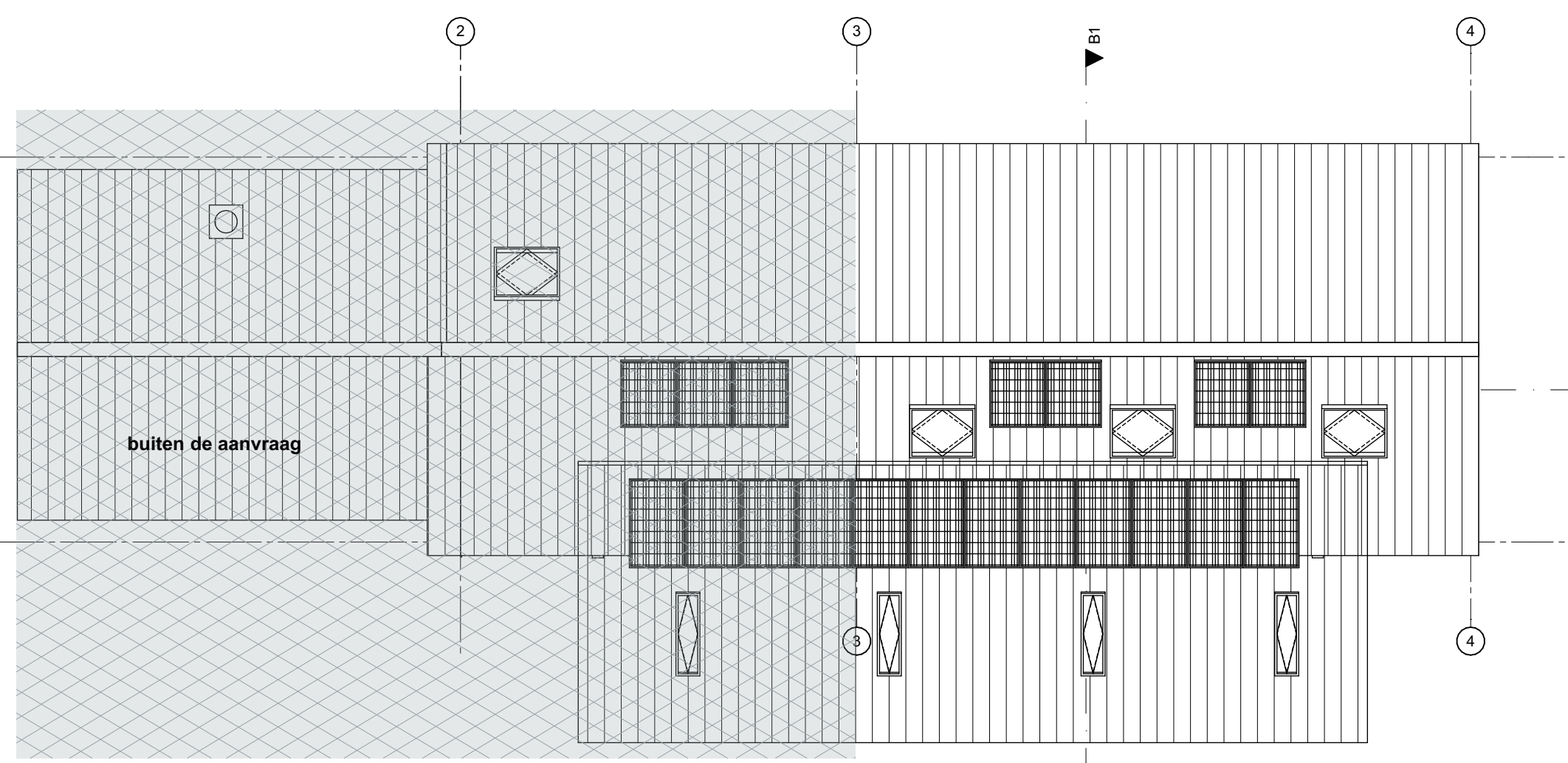
Nok Wierschuur
