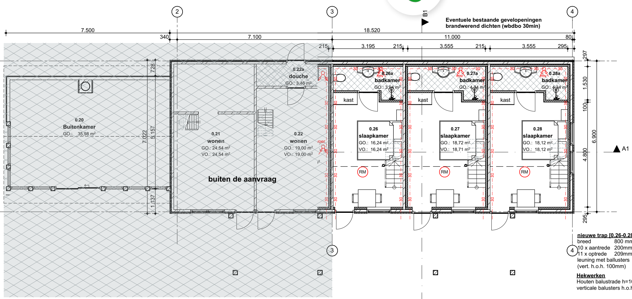
begane grond
