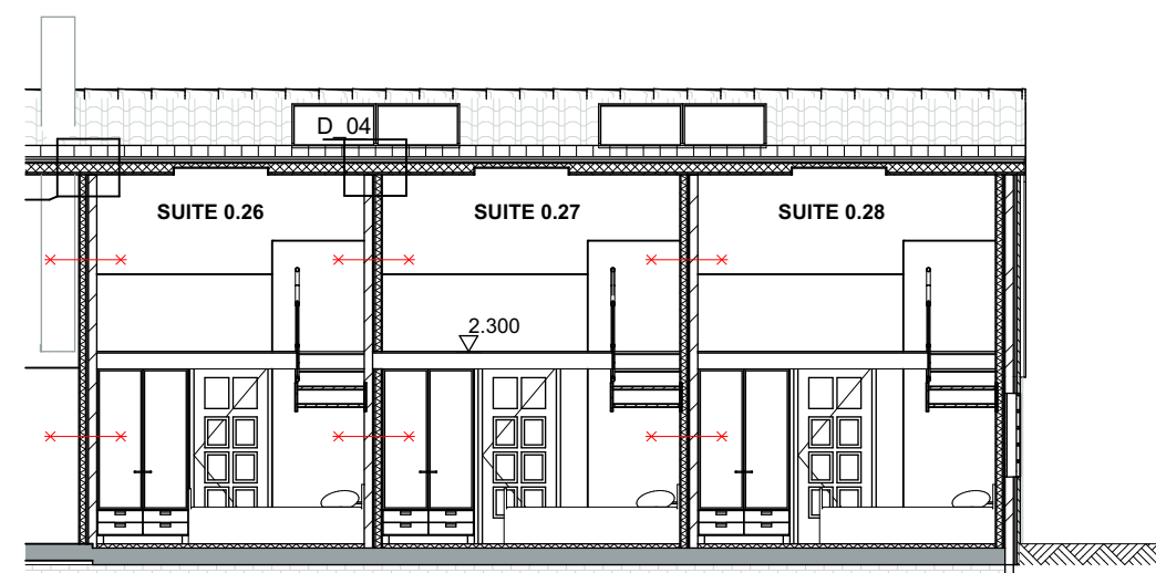
Doorsnede A1-A1
