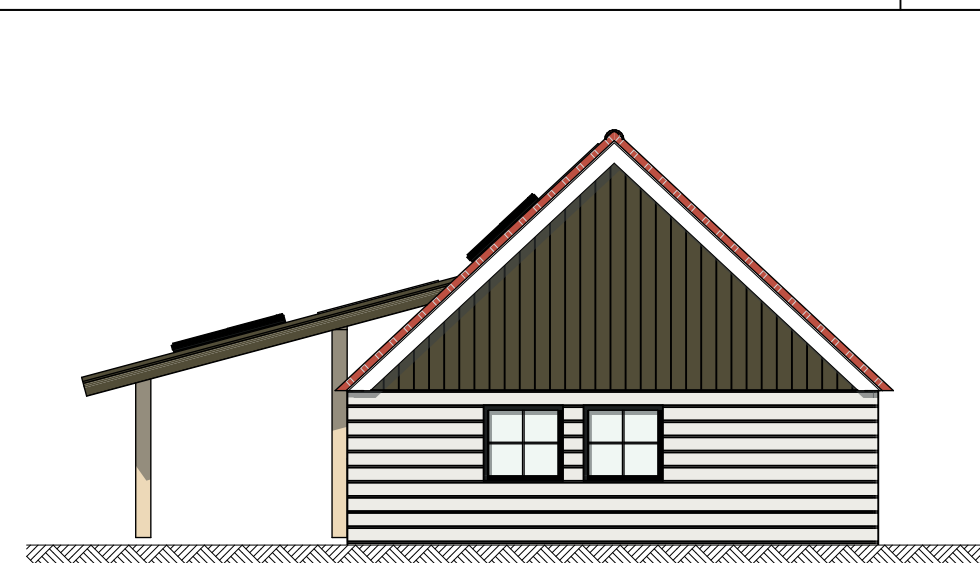
Oostgevel
