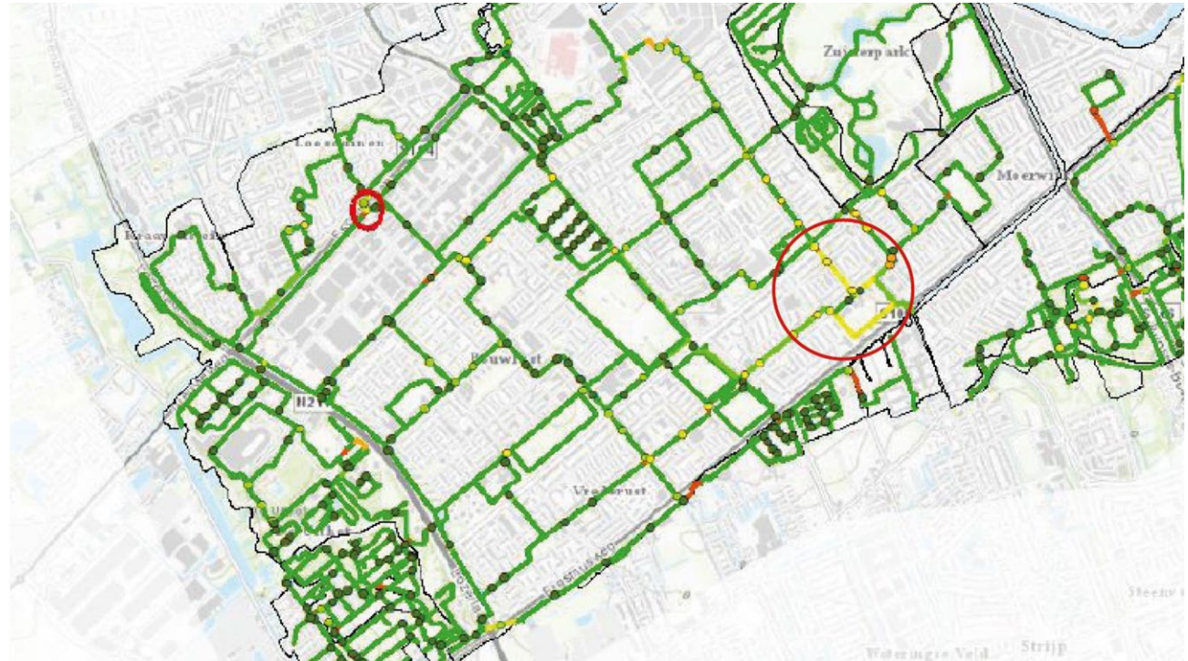
Knelpunten watersysteem (Delfland)
