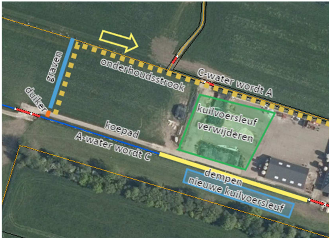
Detail oostelijke kant. Onderhoud vindt plaats vanaf de weg Slappedel
