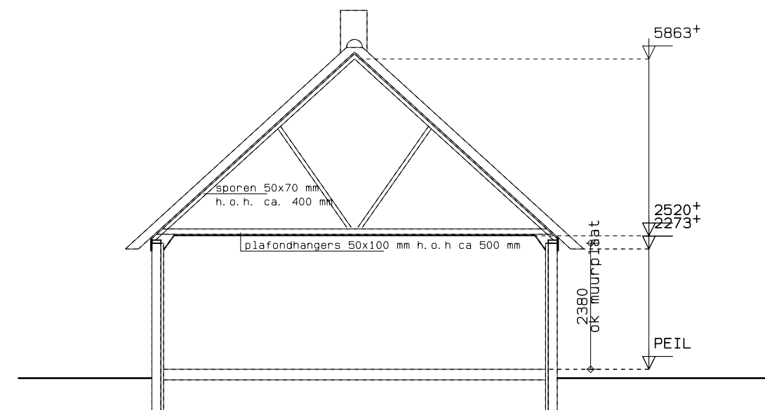
Doorsnede (bestaand)
