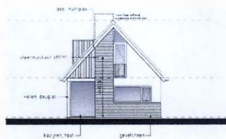
Voorgevel Kavel 5, 7, 9
