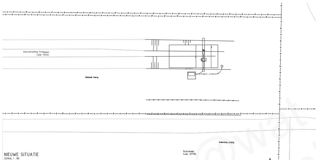
Figuur 6 Uitsnede technische tekening 97188 Stuw Aav 2
