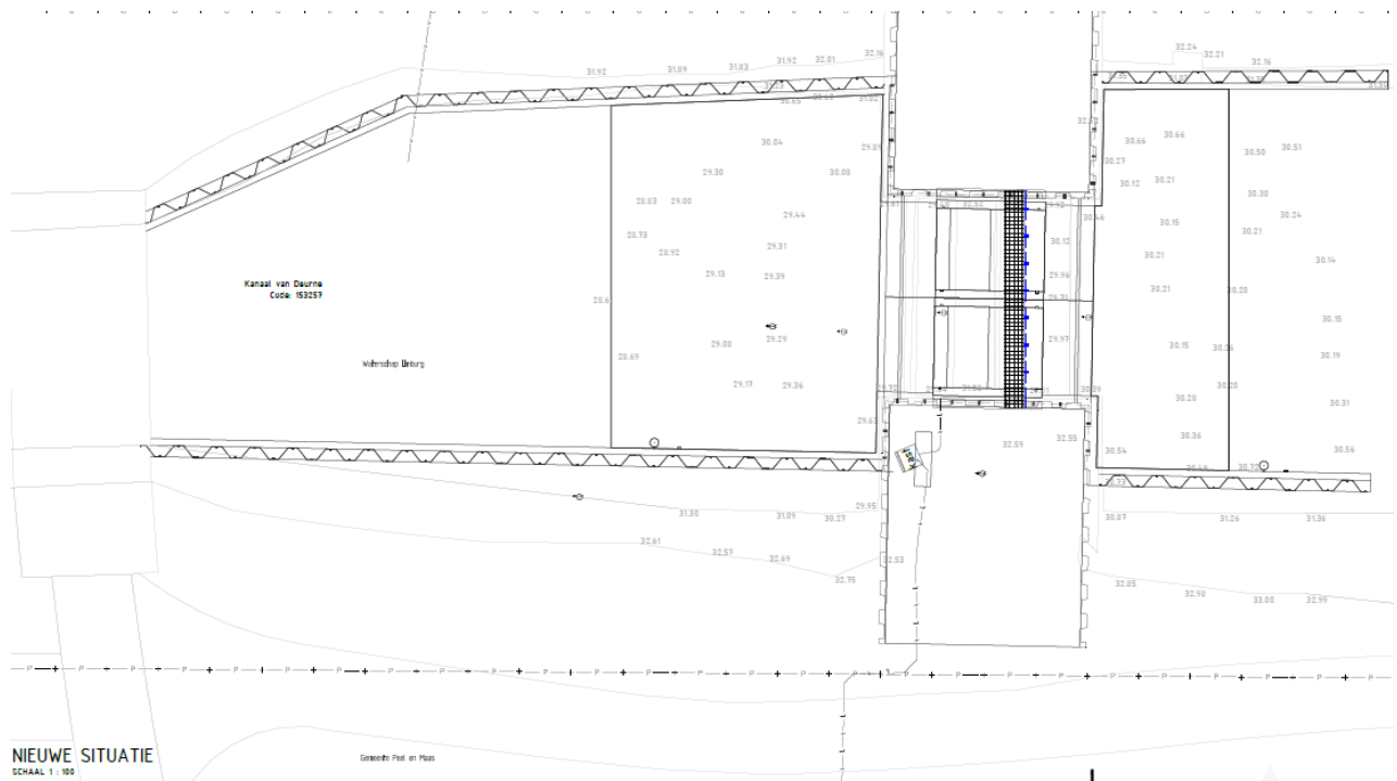
Figuur 15 Uitsnede technische tekening 98176 Stuw Katsberg
