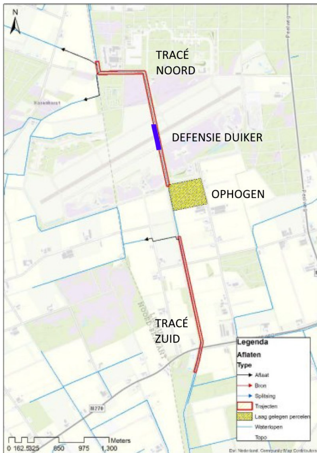
Figuur 16 Overzichtstekening Baggeropgave Defensiekanaal
