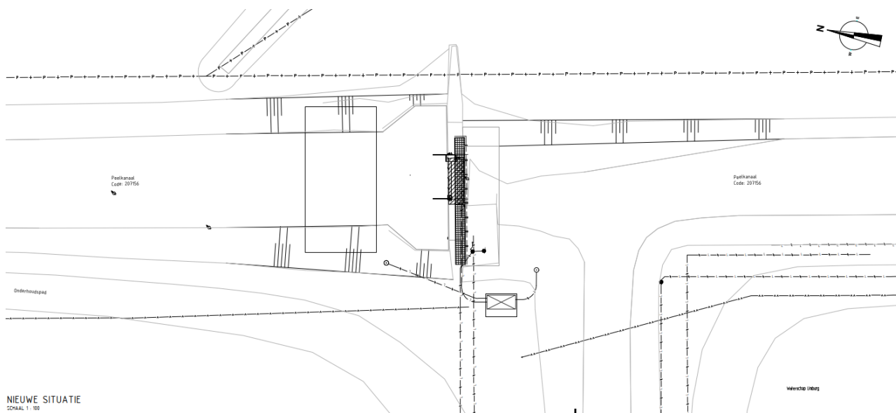
Figuur 9 Uitsnede technische tekening 98249 Klepstuw Kempensberg Noord
