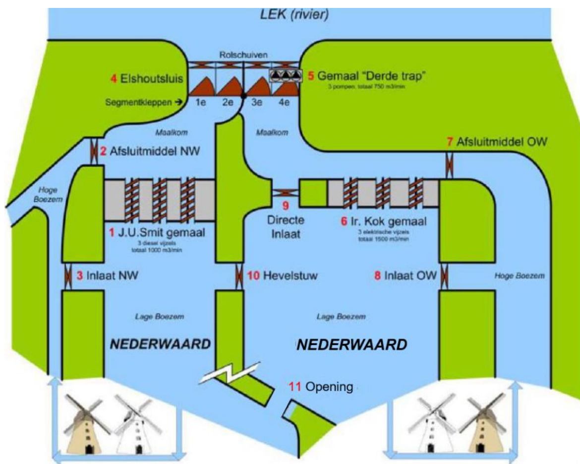
Figuur 3.2: schematische weergave van het nieuwe watersysteem bij Kinderdijk
