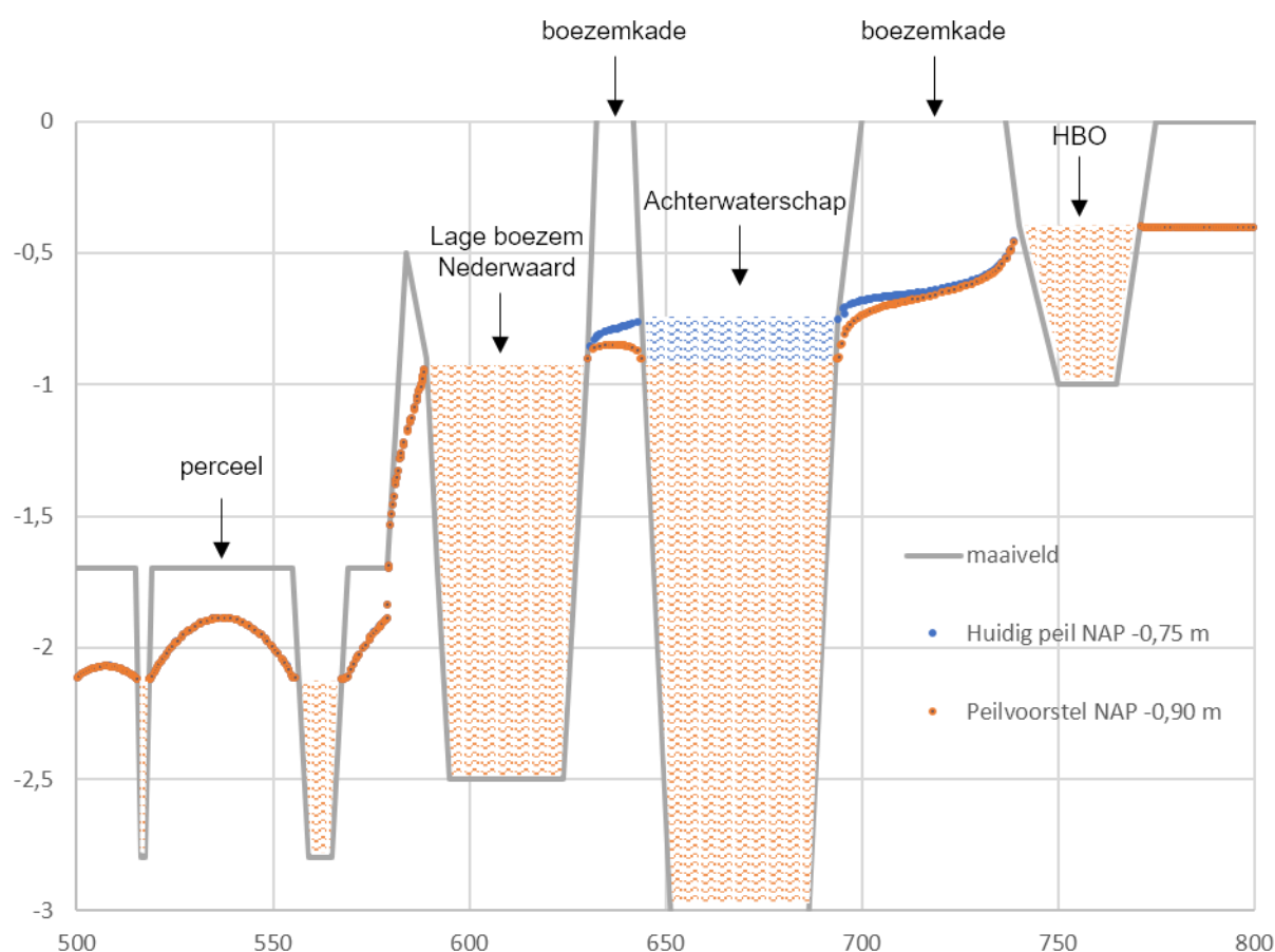
figuur 4.1: effect verlaging boezempeil Achterwaterschap op grondwaterpeil in kades ter hoogte van de HBO (blauw = huidig boezempeil NAP -0,75 m; oranje = boezempeil NAP -0,90 m) [ref. 7]
