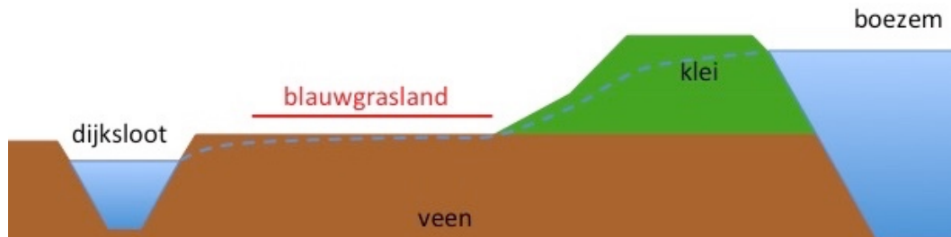
Figuur 4 Profiel dijktaalud op plaatsen met blauwgrasland. Er zijn slechts enkele dm diepe boringen uitgevoerd, dus de grondwaterstand en bodem zijn slechts indicatief. In dit profiel ontbreekt (buitendijks) boezemland.
