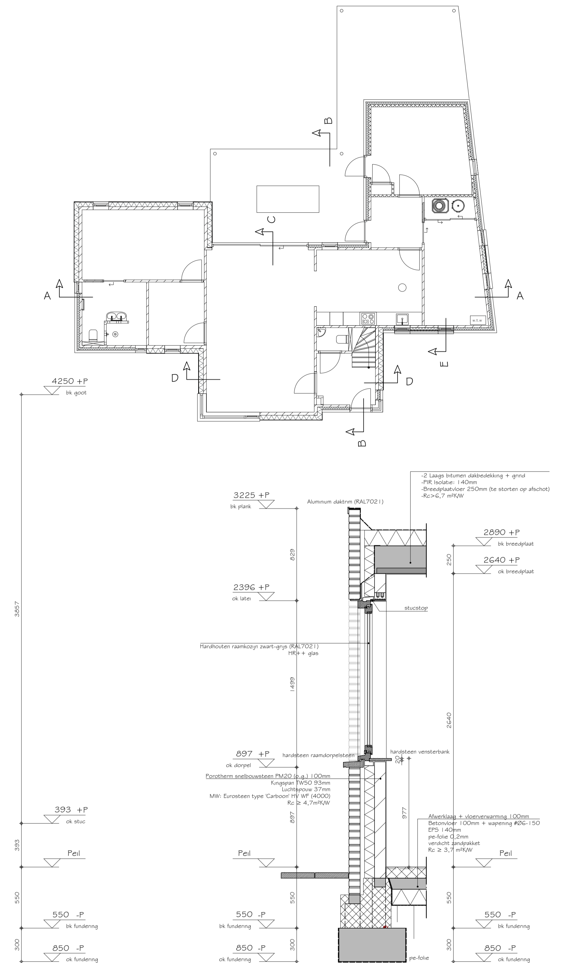
DOORSNEDE E
