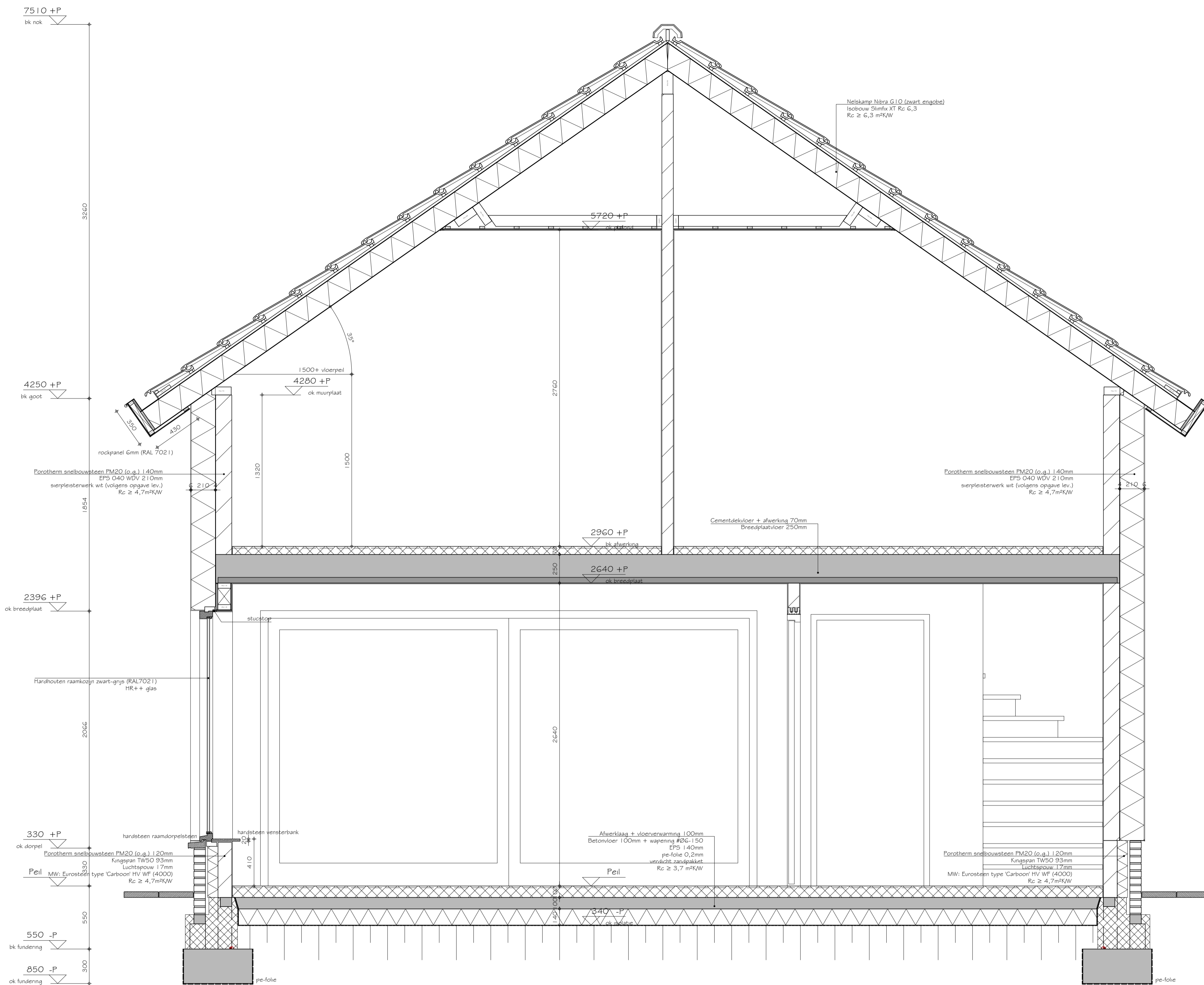
DOORSNEDE D-D
