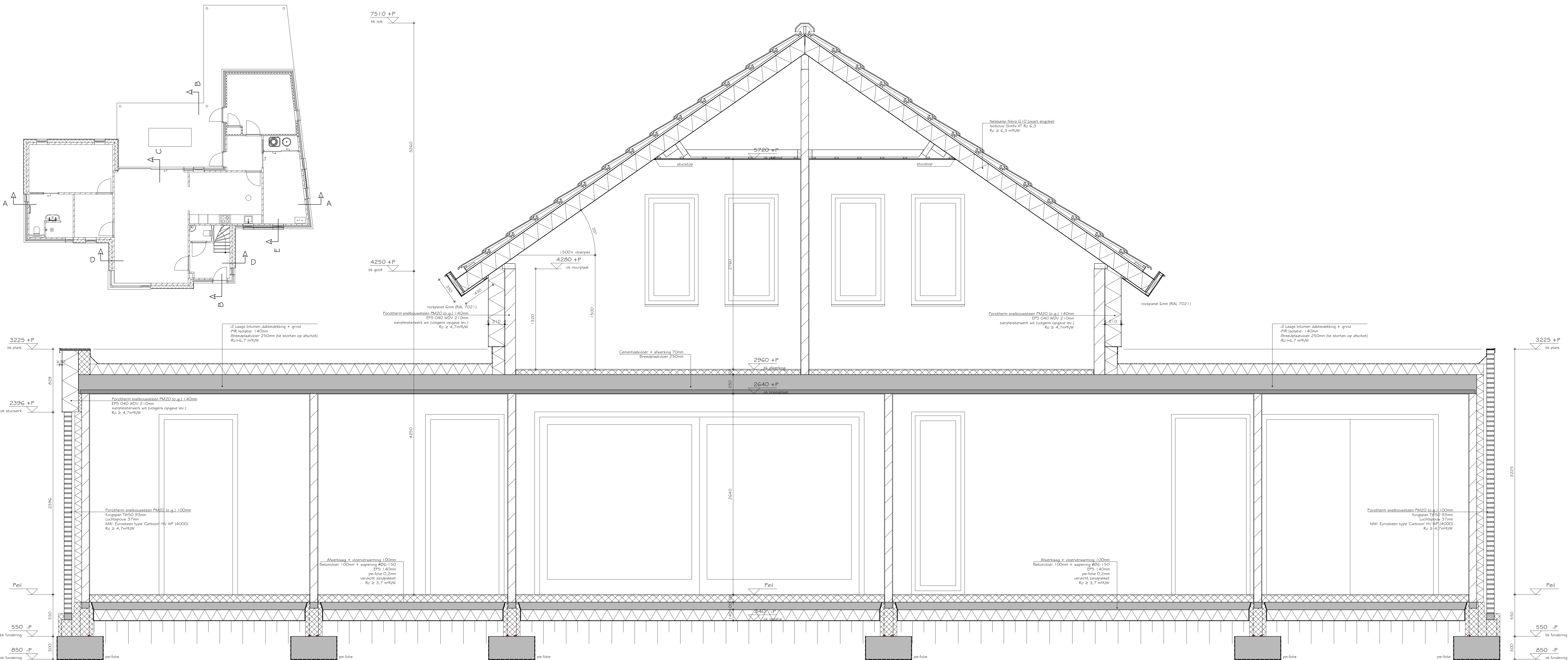
DOORSNEDE A-A
