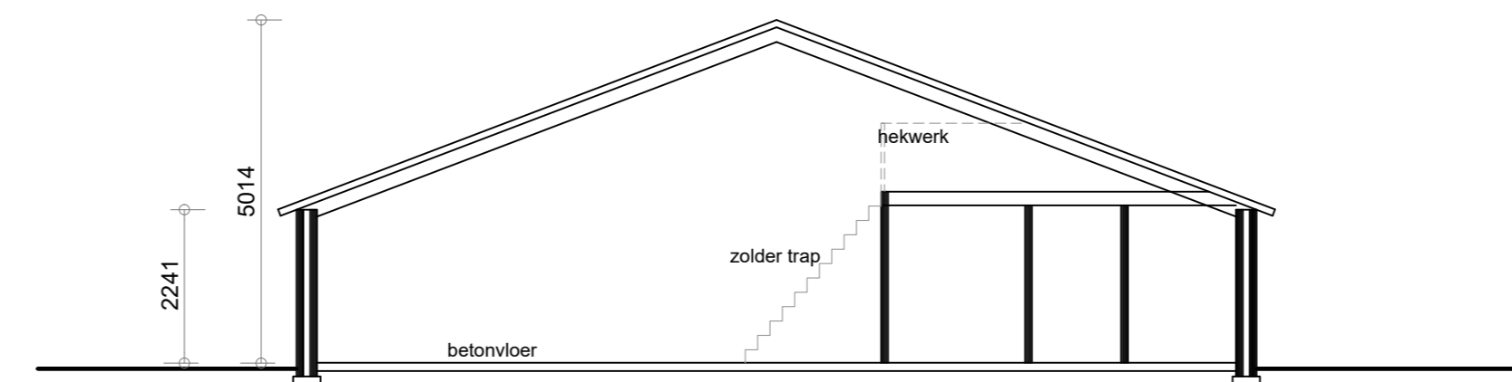
- Doorsnede C - C -
