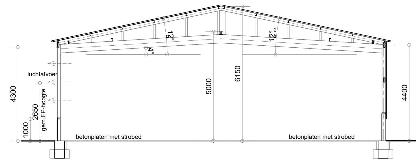
- Doorsnede A - A -
