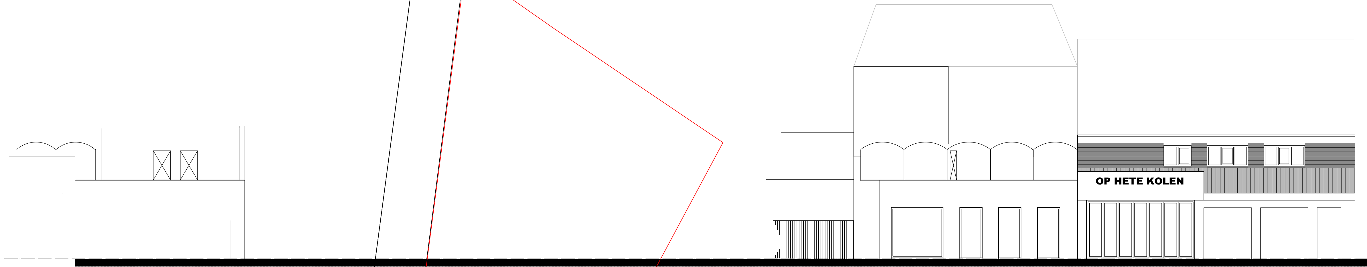
RECHTER-ZIJGEVEL TOESTAND BESTAAND
