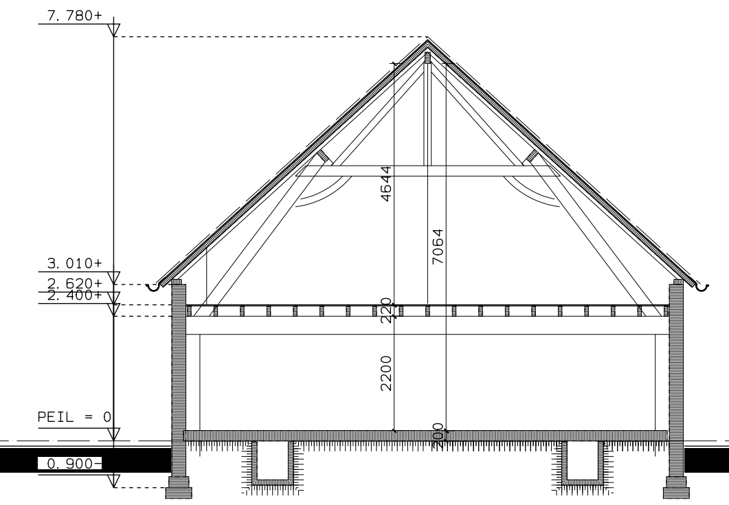
doorsnede
