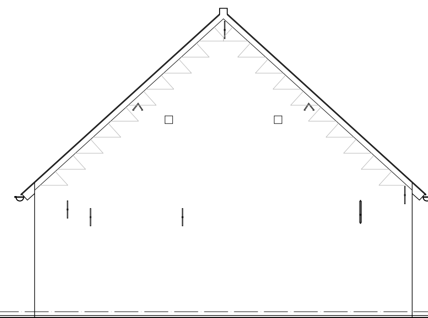
noordoostgevel
