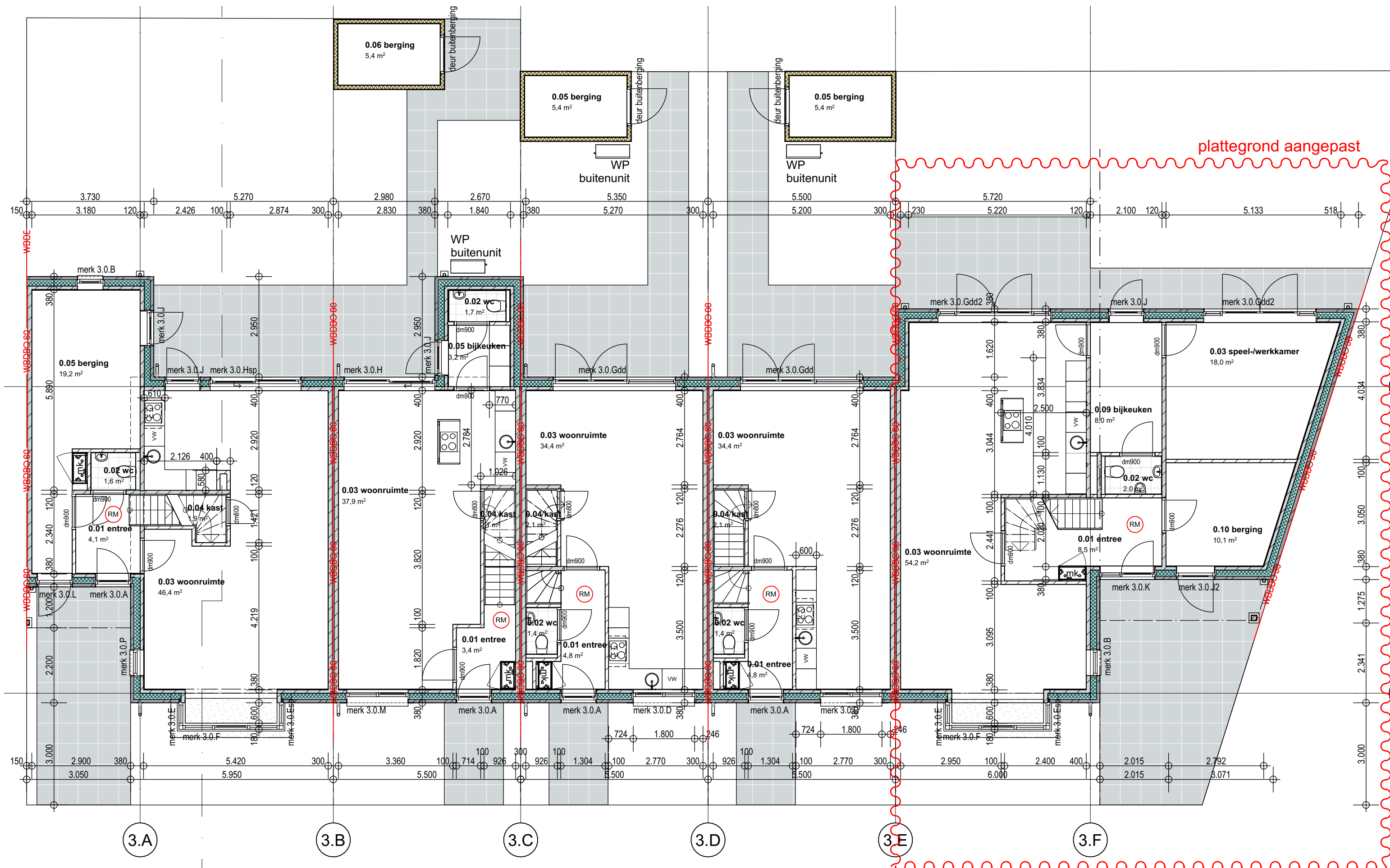
0 begane grond 1:100
