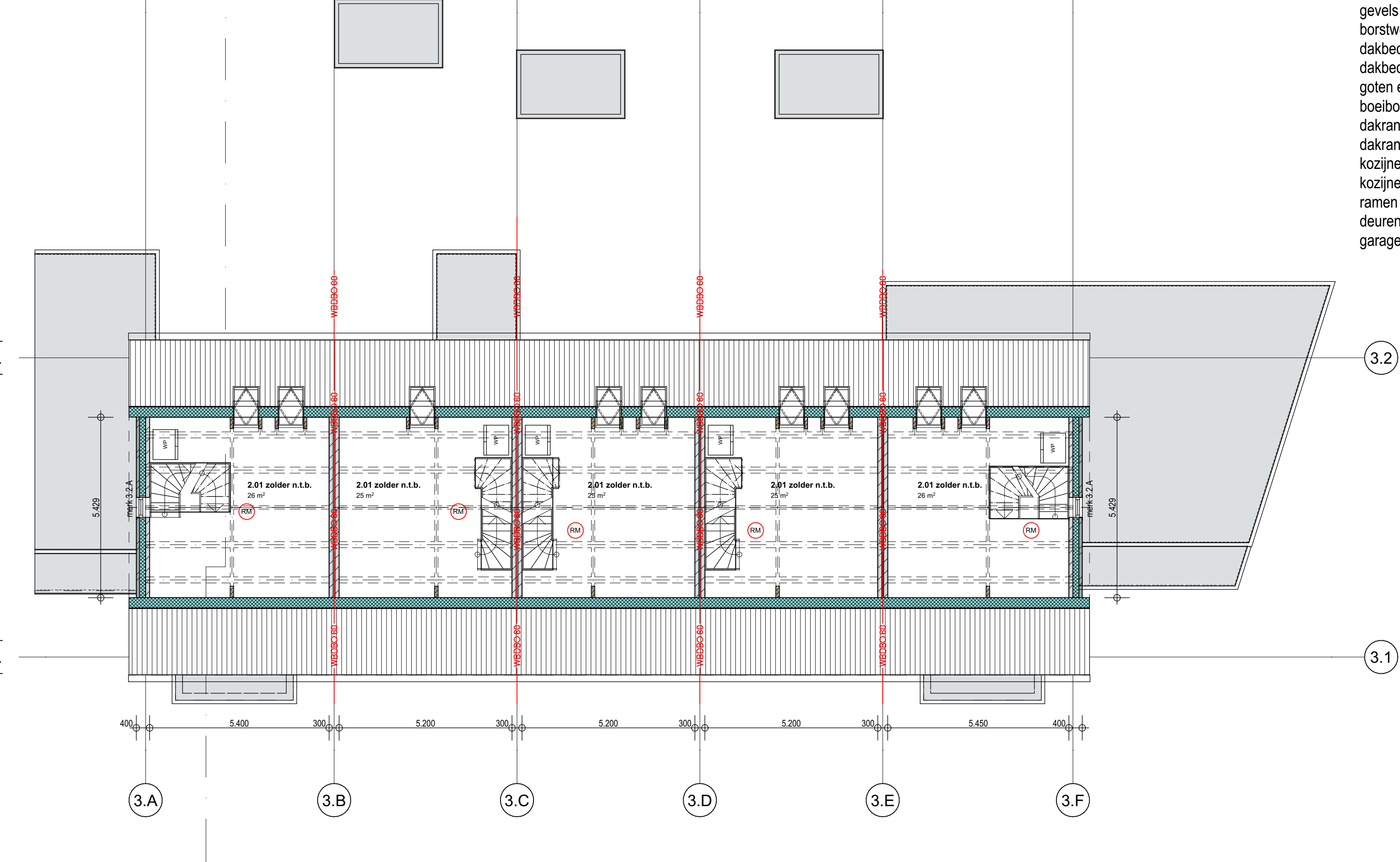
2 tweede verdieping 1:100
