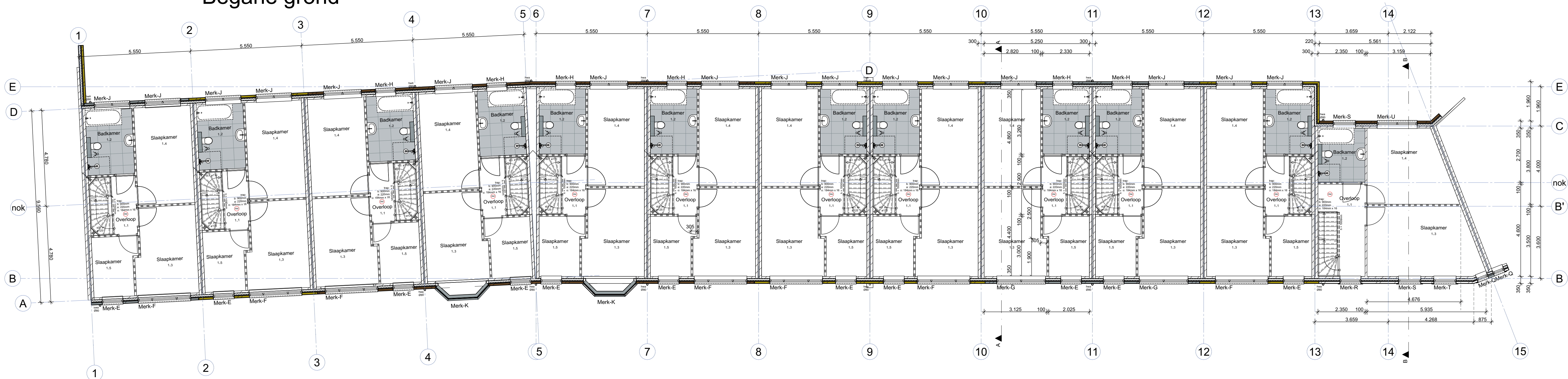
1e verdieping 2940+P
