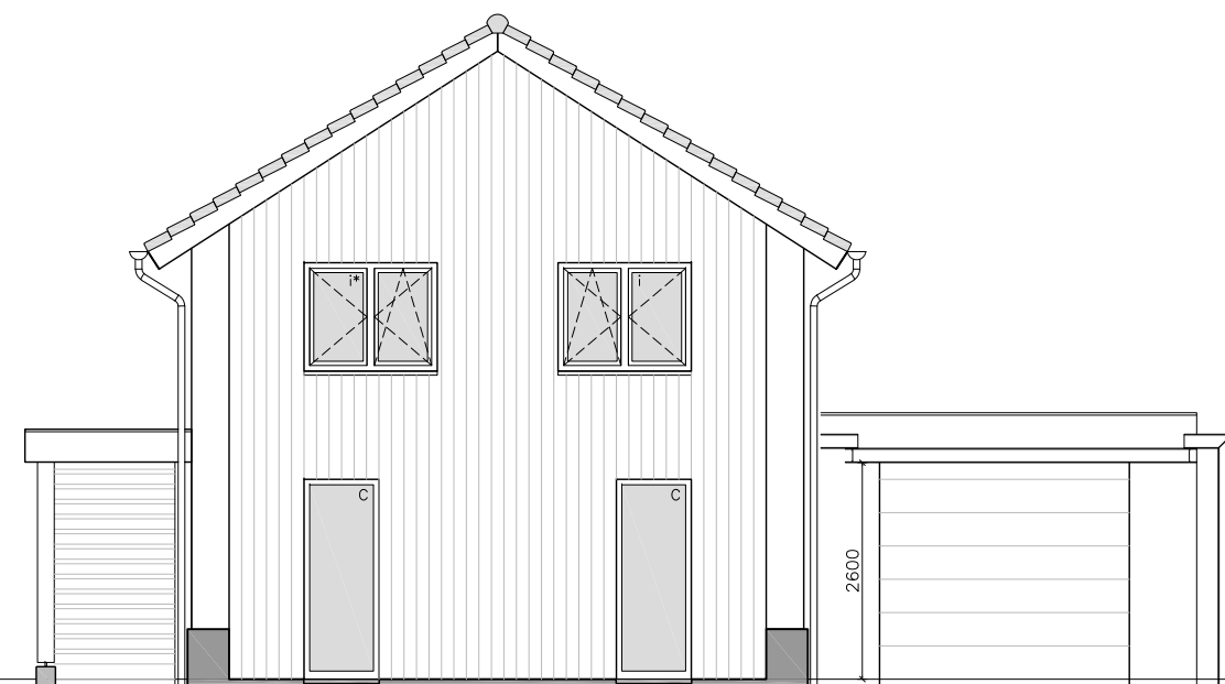
VOORGEVEL - nieuw schaal 1:100
