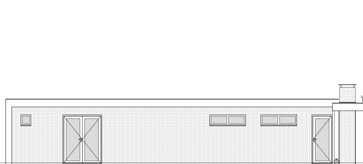
LINKERZIJGEVEL - nieuw schaal 1:100
