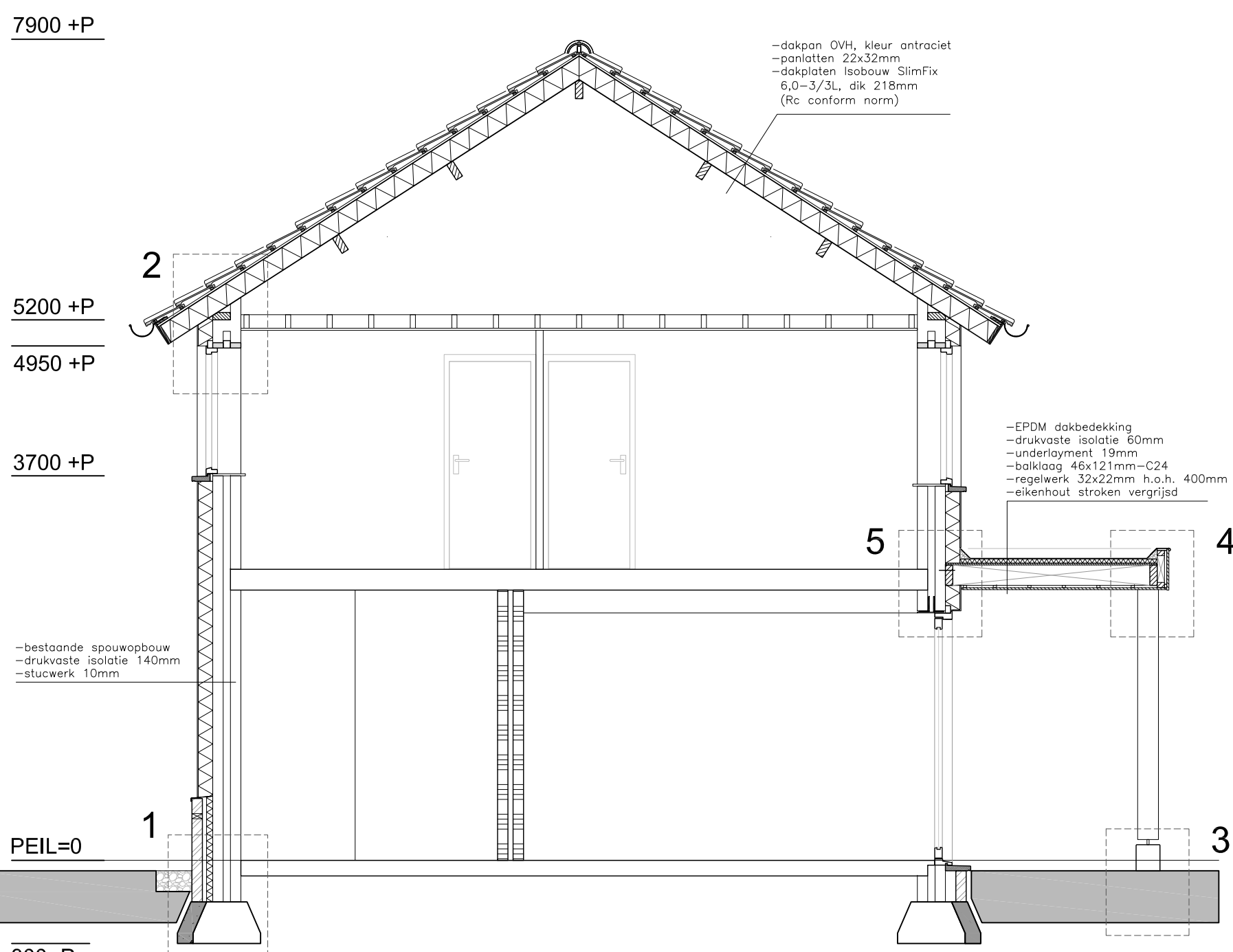
DOORSNEDE A-A - nieuw schaal 1:50
