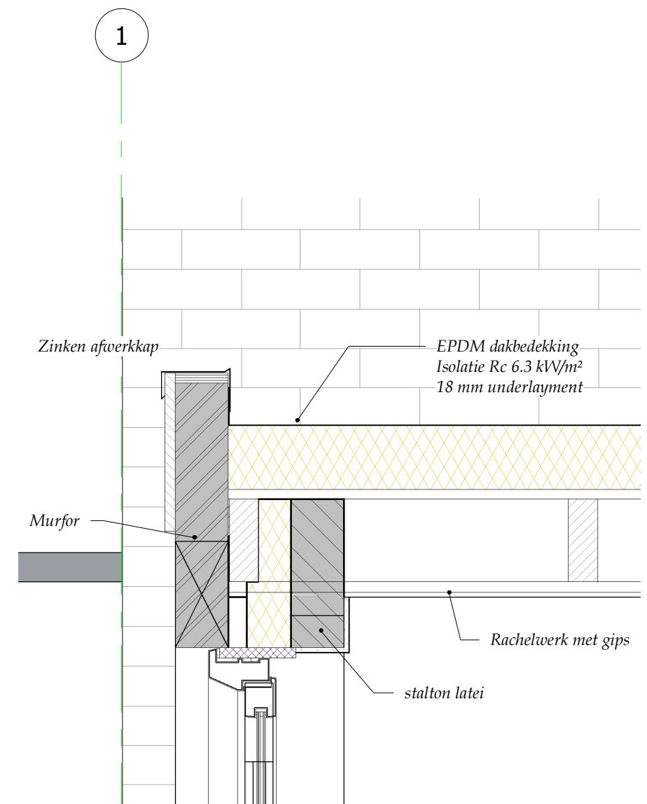
3 B/B - Callout 2 1 : 10
