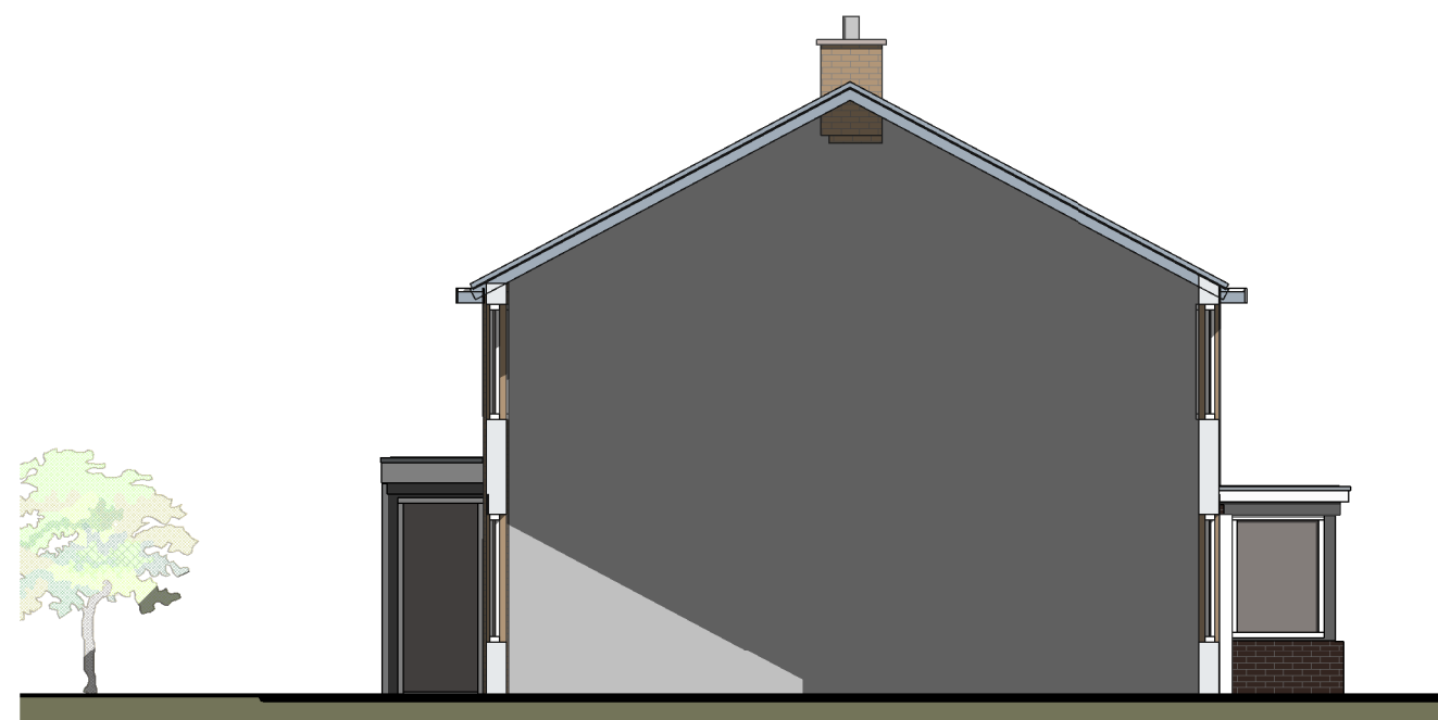
1 Linkerzijgevel Nieuw 1 : 100
