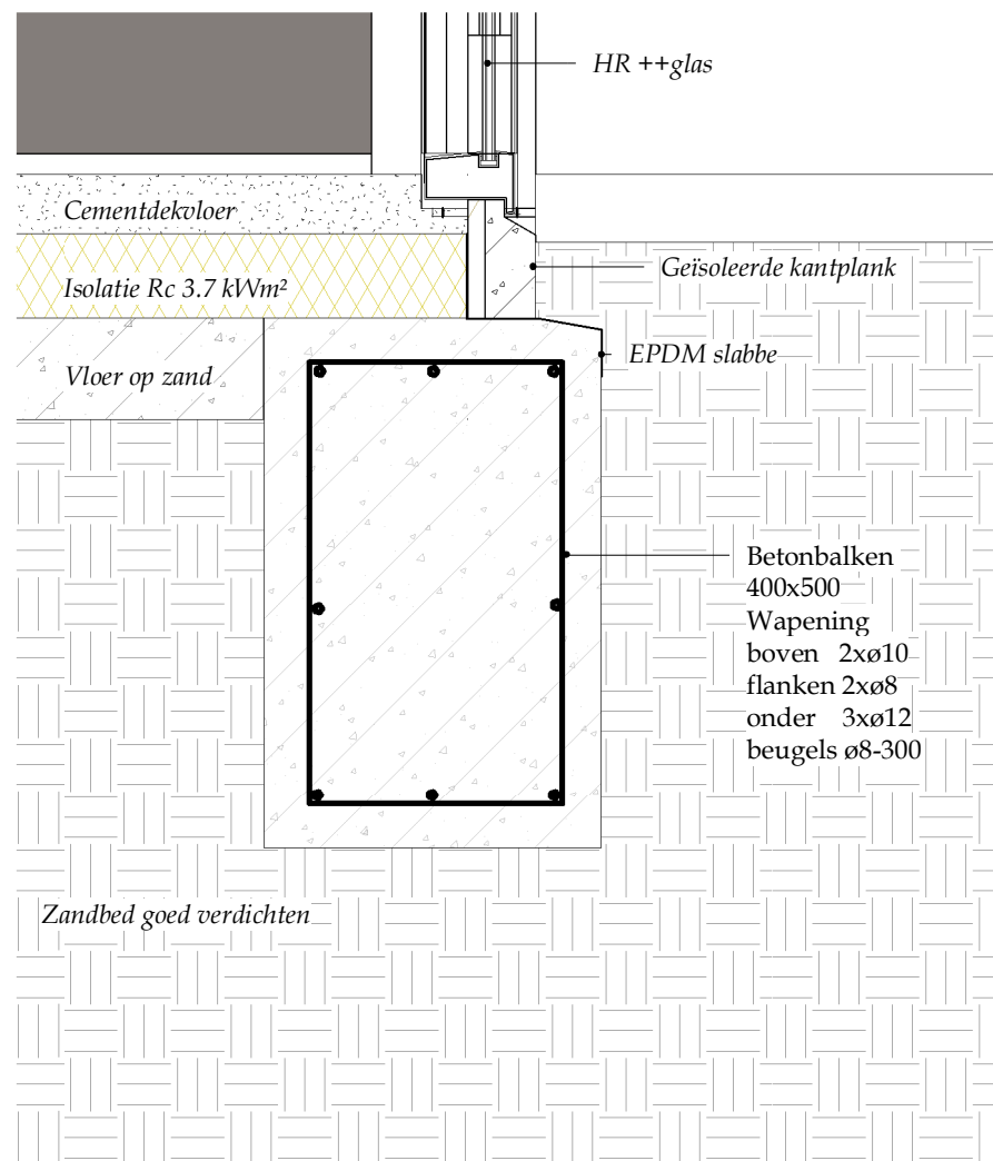
2 B/B - Callout 1 1 : 10
