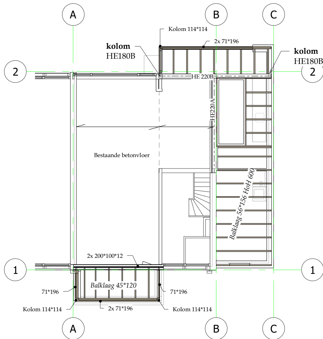
1 Balklaag 1 : 100
