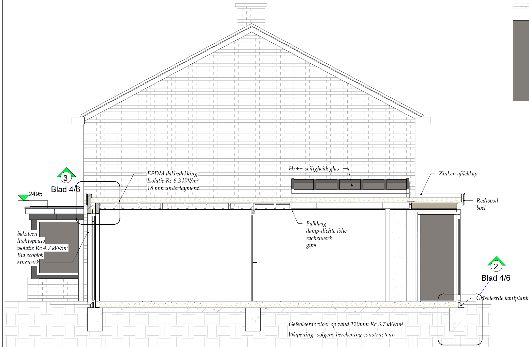
1 Doorsnede B/B 1 : 50
