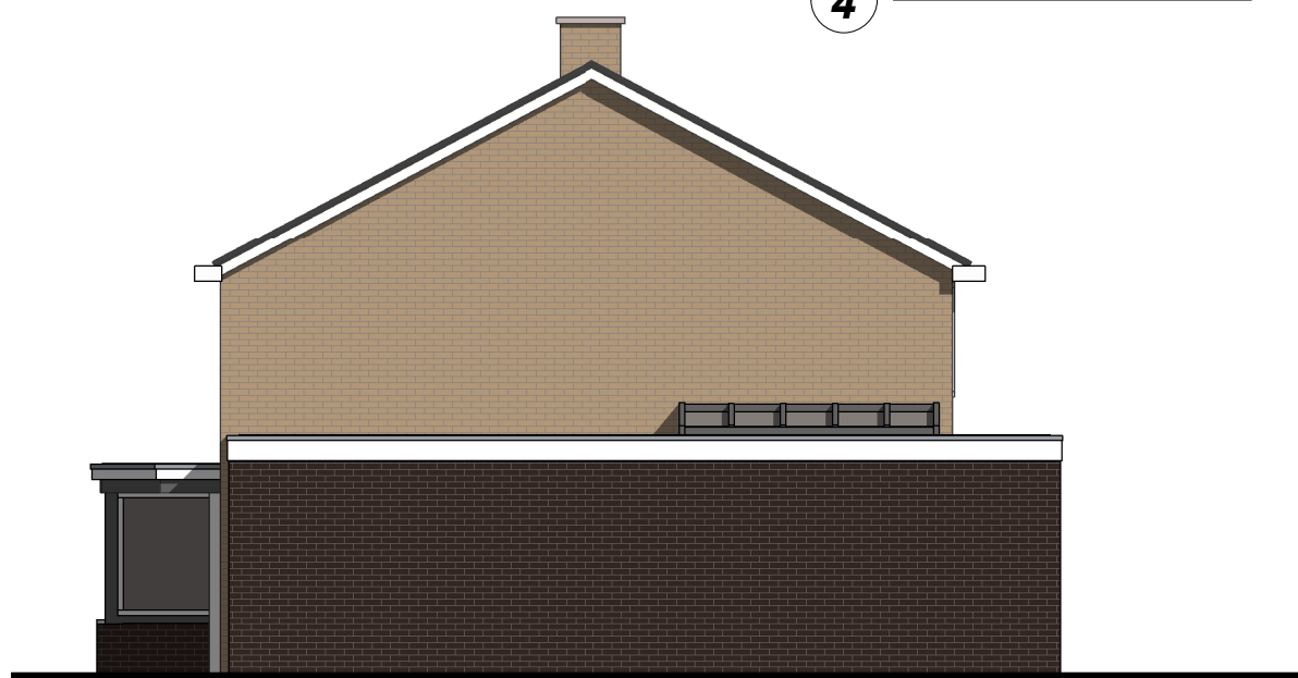
3 Rechterzijgevel Nieuw 1 : 100
