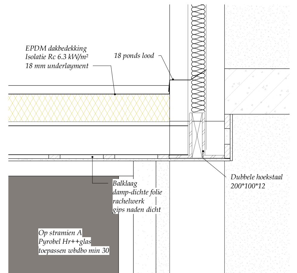
2 C/C - Callout 3 1 : 10
