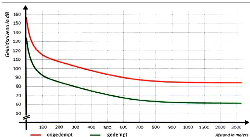
Afbeelding 2: Relatie tussen geluidsniveaus en de afstand voor een geweer zonder en met demper (bron: Jagd mit schalldämpfer, [redacted], 2014).
