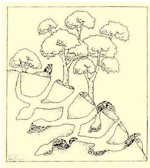
Figuur 4: Schematische voorstelling van een dassenburcht (bron: dasenboom.nl)
