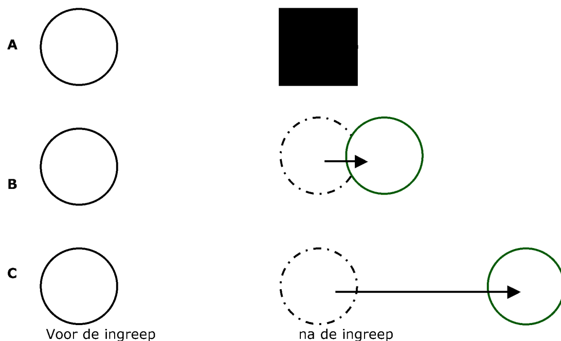
Figuur 8: behoud gunstige staat van instandhouding. Links de situatie voor de ingreep, rechts de situatie na de ingreep.
