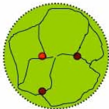
Figuur 6: Schematische voorstelling van een dassenterritorium (groen) met een hoofdburcht (rood) en bijburchten of vluchtpijpen (bruinrood) en veel gebruikte wissels (lijnen)
