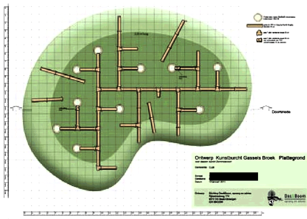
Figuur 9: voorbeeld van een ontwerp van een kunstburcht (bron: dasenboom.nl). In dit geval is gebruikgemaakt van gresbuizen voor de pijpen en op de kop geplaatste bijpassende ronde systeempotten. De terp is 2,5 meter hoog en circa 30 meter breed en er zijn twee ontluuchtingspijpen aangebracht. Het ontwerp van de kunstburcht is afhankelijk van dat wat verloren gaat.
