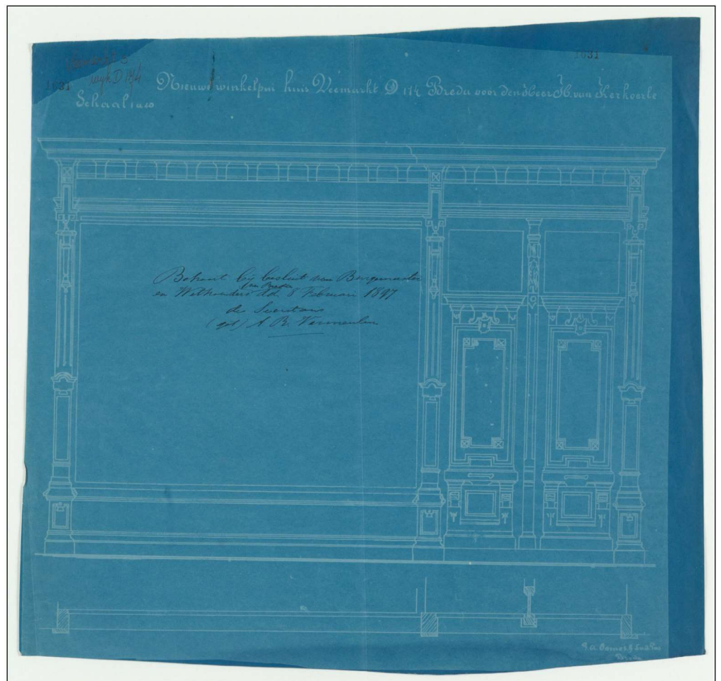
Afb. 61: Wijziging van de onderpui in 1897. Zie afb. 8. [Stadarchief Breda]
