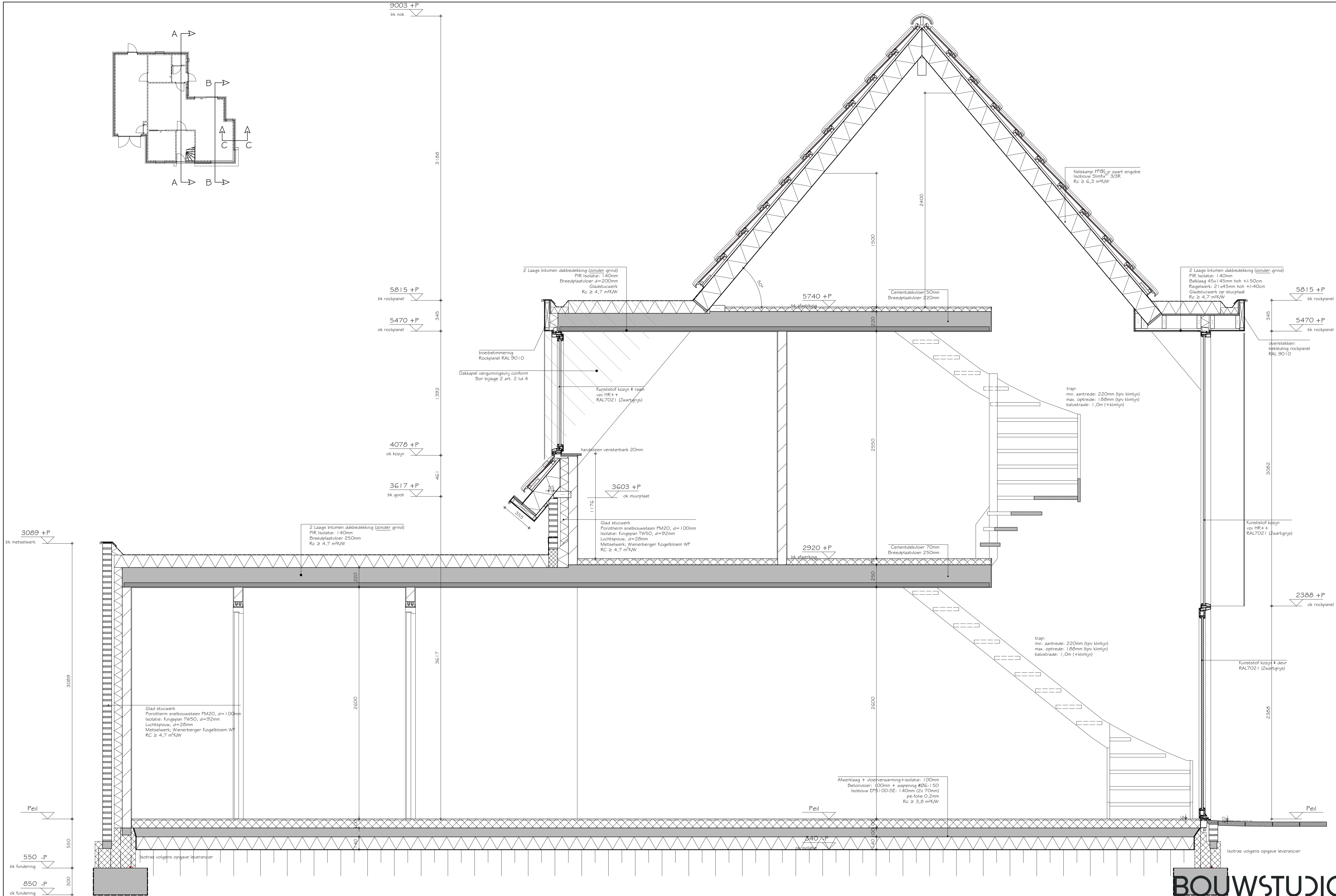
DOORSNEDÉ A-A
