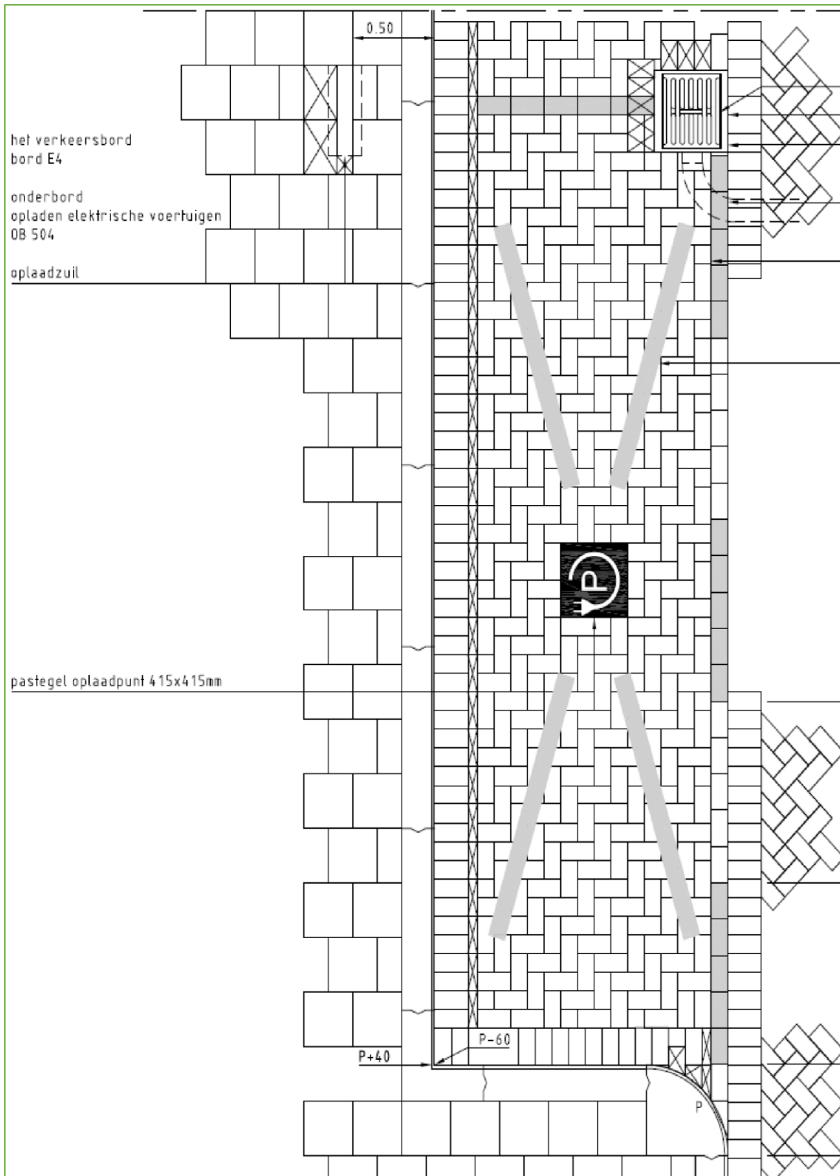
Figuur 3: Inrichting laadvakken bij langsparkeren
