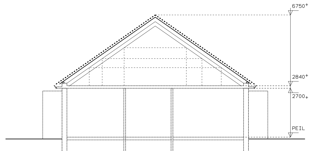
Doorsnede (bestaand)
