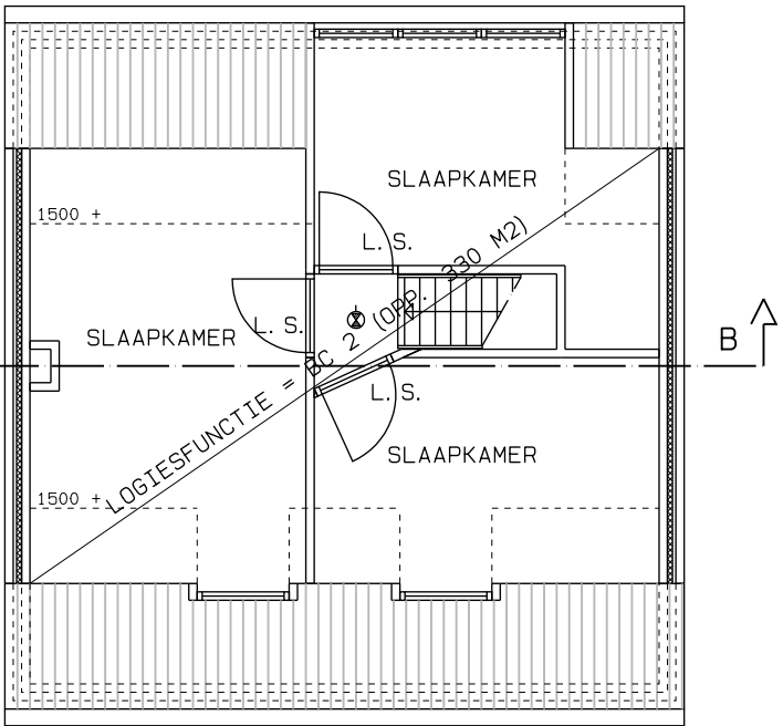
2e Verdieping (blijft ongewijzigd)
