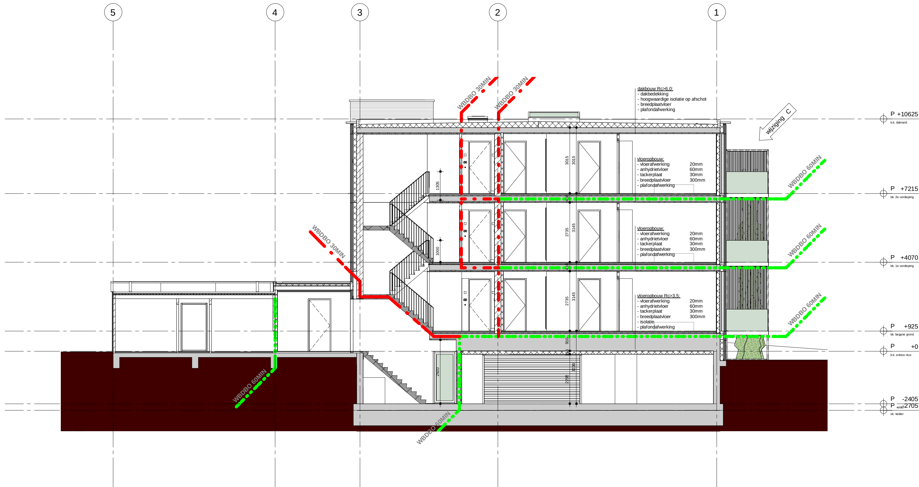
doorsnede E
