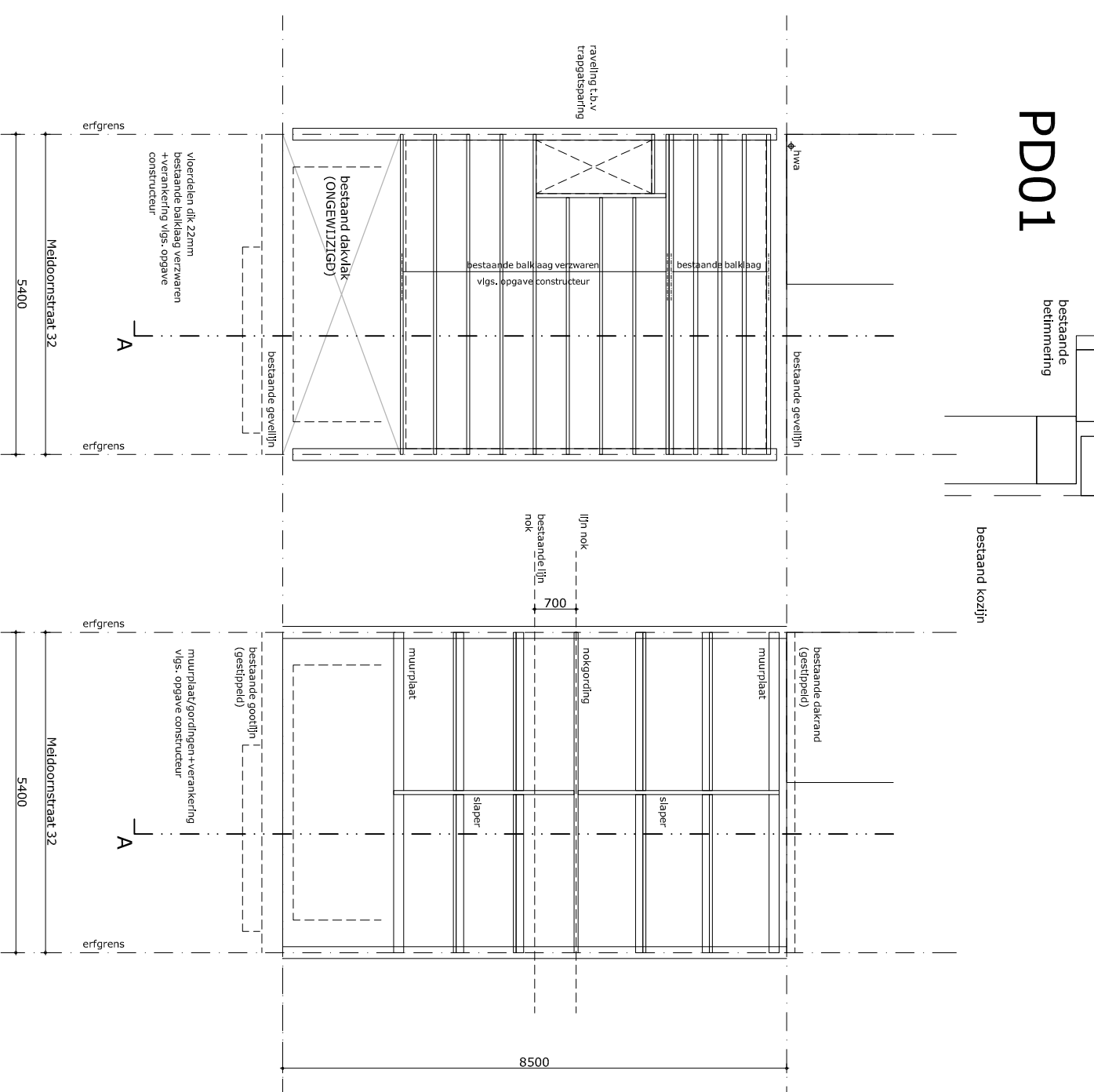
viëringvloer NIEUWE TOESTAND
