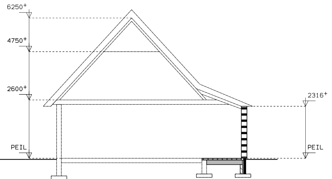
Doorsnede (bestaand)
