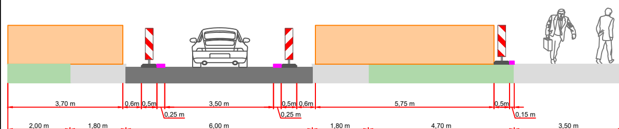
Dwarsdoorsnede A-A
