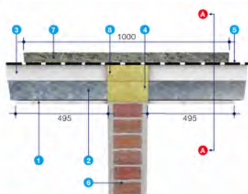
Dwarsdoorsnede 60 min.
