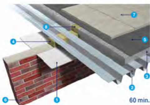
Dwarsdoorsnede 60 min.
