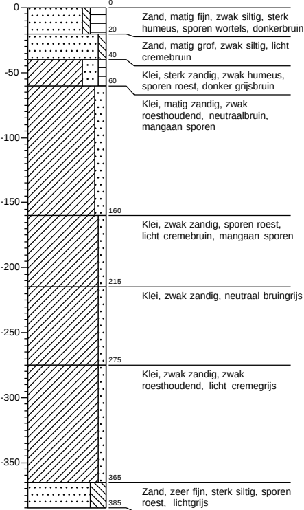
Boring A11
