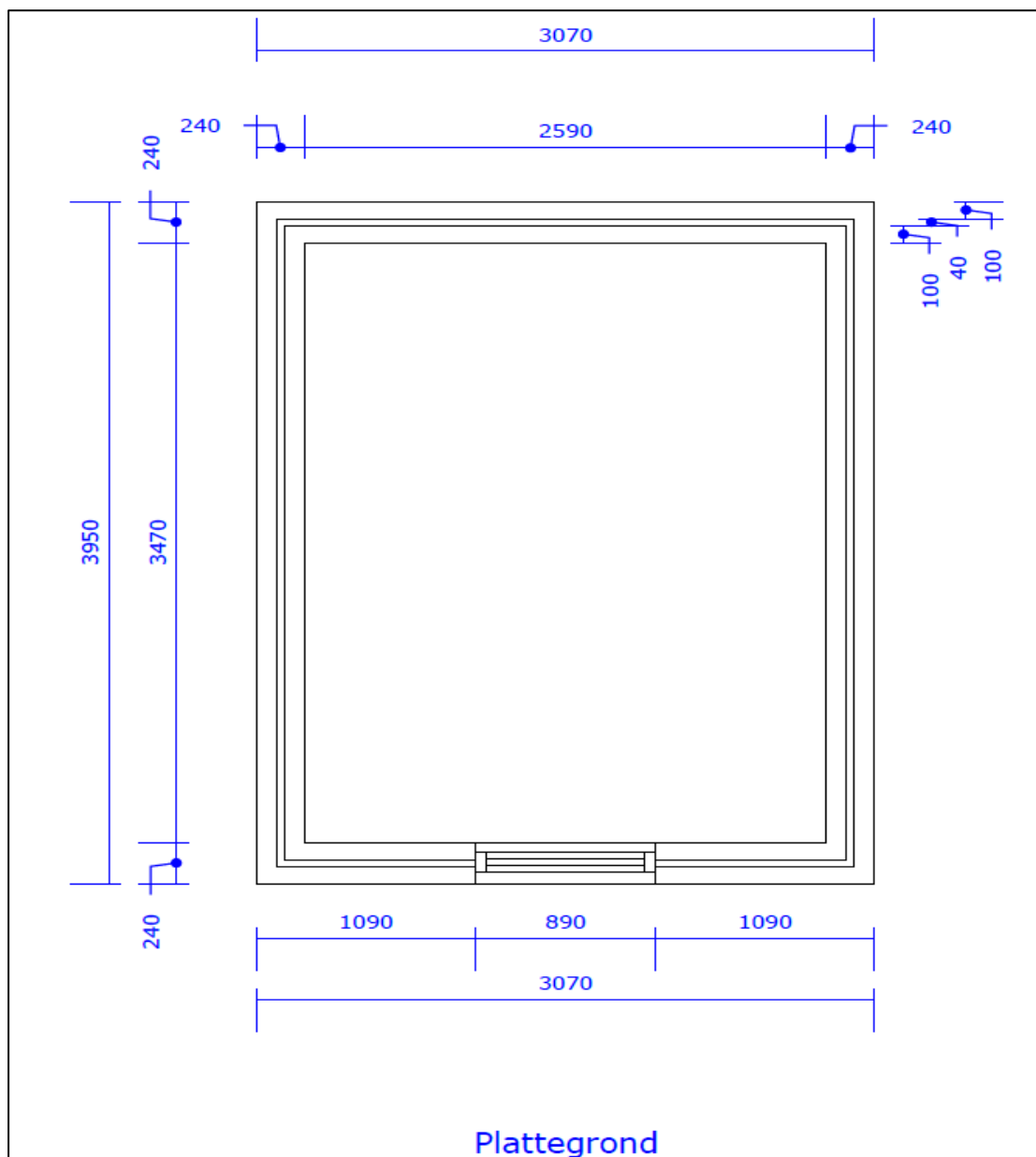
Figuur 3. Een overzicht met plattegrond van de vleermuistoren. De toren dient conform deze maten gebouwd te worden. Naast deze detailfoto van de plattegrond, dient de toren gebouwd te worden conform de beschreven maatvoering (fundering, dak, overstek, spouw etc.) in het bij de aanvraag gevoegde document 'Toren te Eibergen, opdrachtgever Faunus Nature Creations' (Bouwbedrijf W. Nijhuis, d.d. 15 december 2021) (documentnummer: 03604410).
