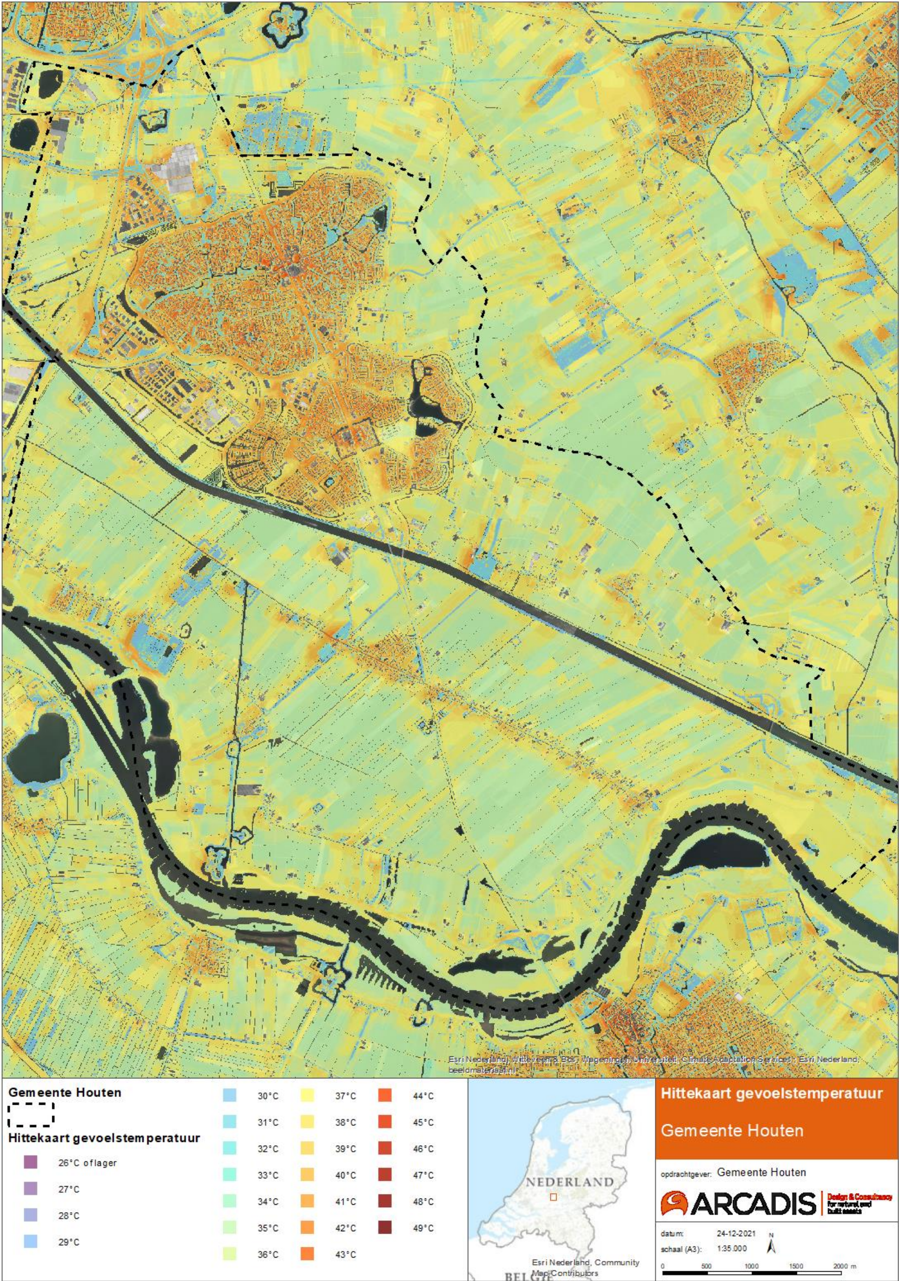
B.2.a: Hitte - Gevoelstemperatuur (bron: Stichting CAS; klimaateffectatlas)
